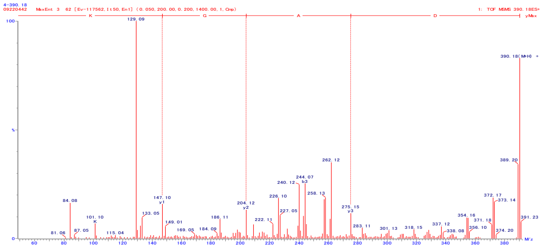
図 17. DAGK の 2 級質量スペクトル
