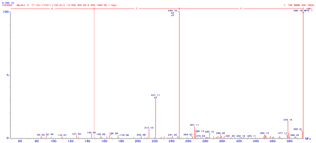
図 42. FTE の 2 級質量スペクトル
