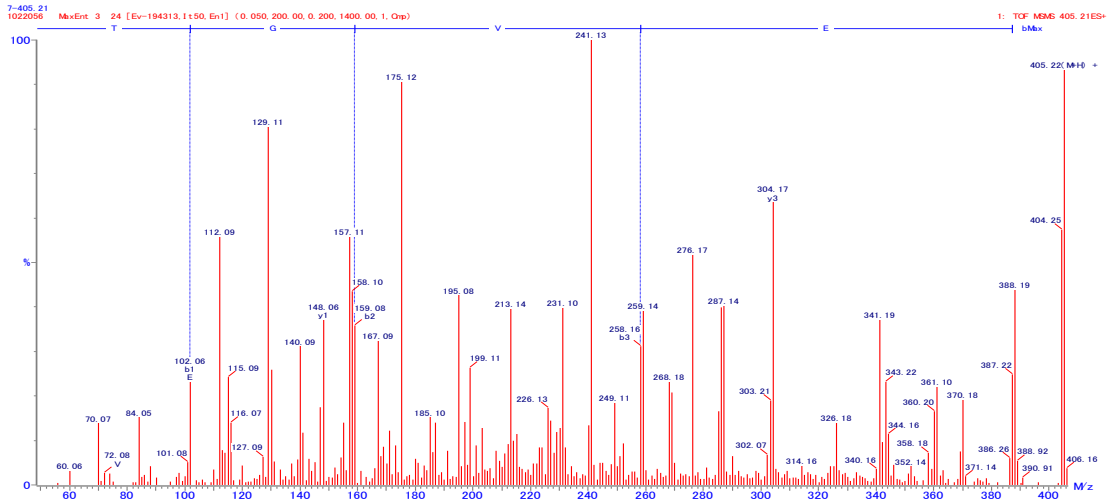
図 32. TGVE の 2 級質量スペクトル
