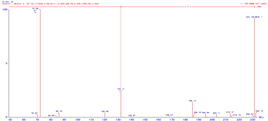
図 55. VL の 2 級質量スペクトル
