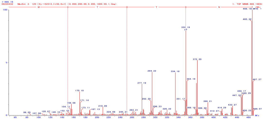
図 2. NTM の 2 級質量スペクトル
