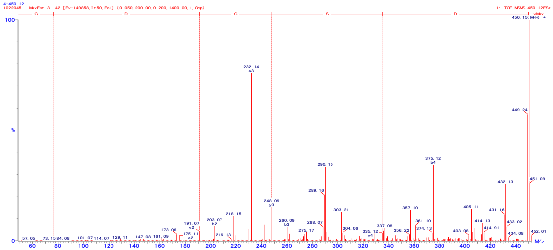
図 23. DSGDG の 2 級質量スペクトル
