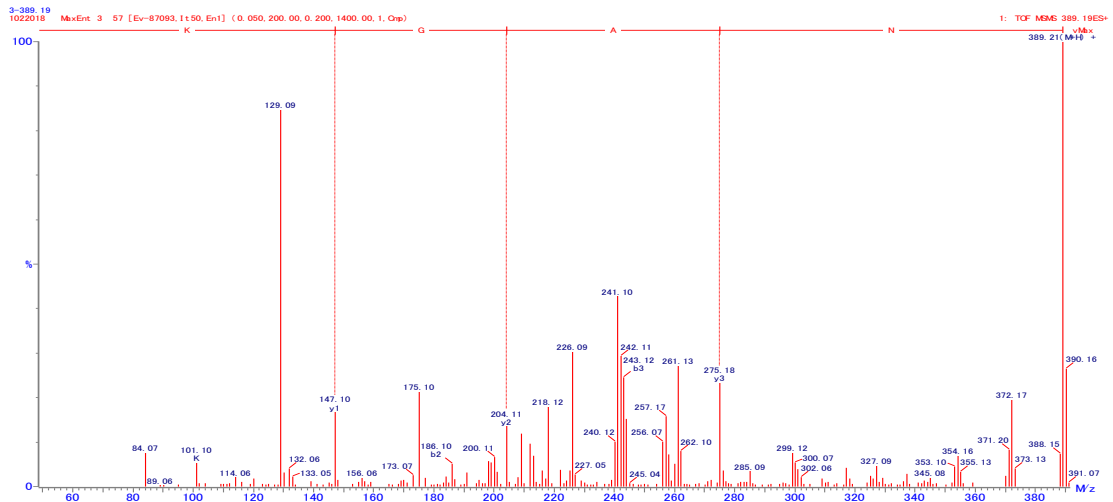
図 12. NAGK の 2 級質量スペクトル
