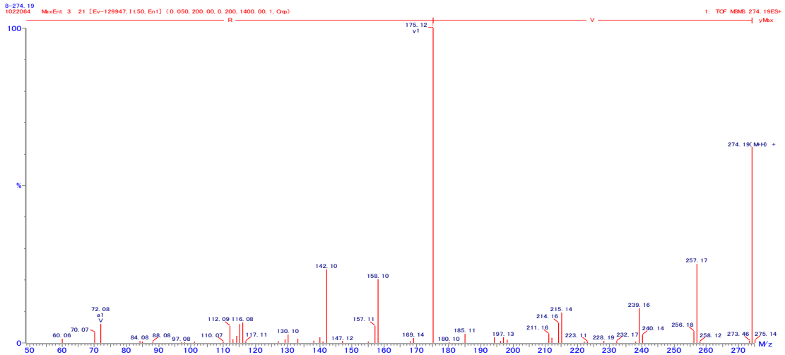
図 35. VR の 2 級質量スペクトル
