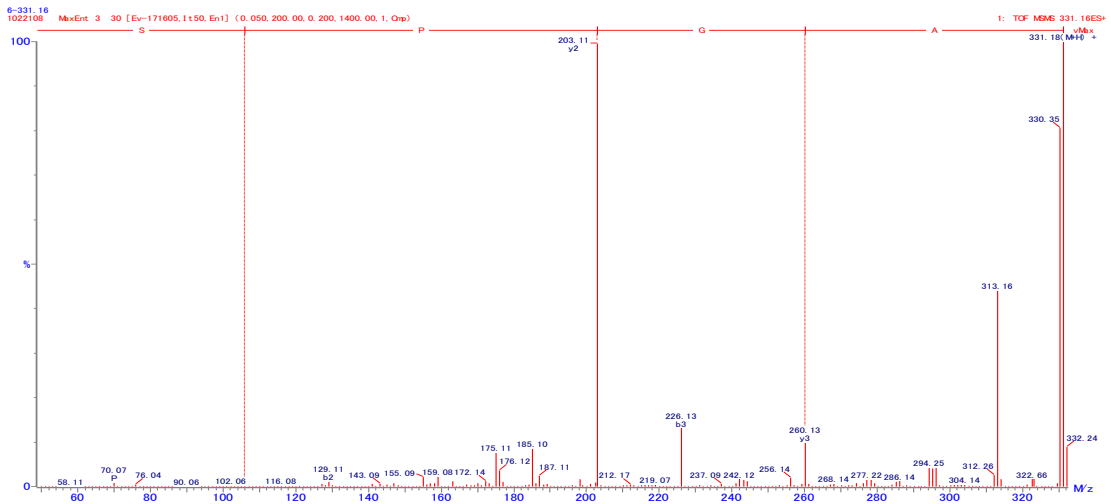
図 24. AGPS の 2 級質量スペクトル
