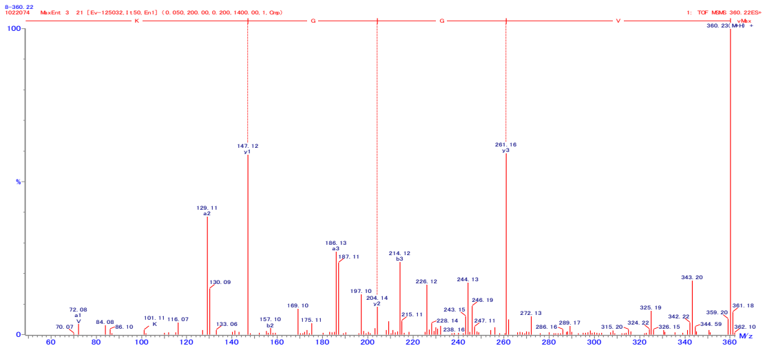
図 39. VGGK の 2 級質量スペクトル
