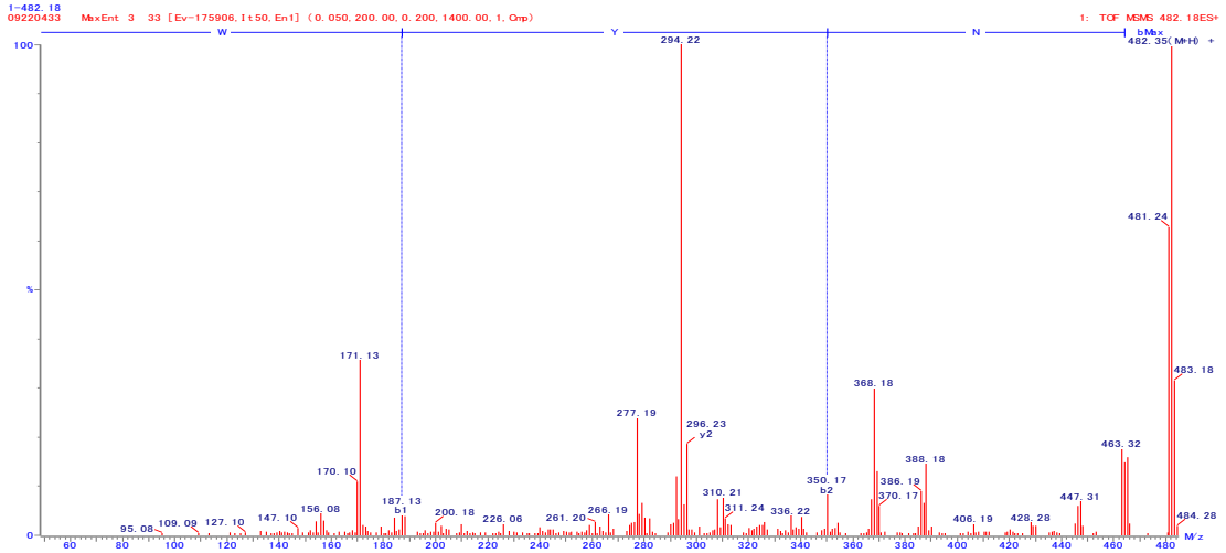
図 1. WYN の 2 級質量スペクトル
