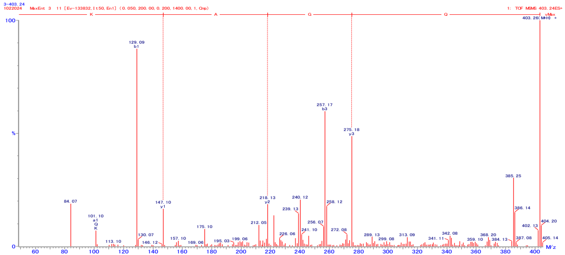
図 14. QGAK の 2 級質量スペクトル
