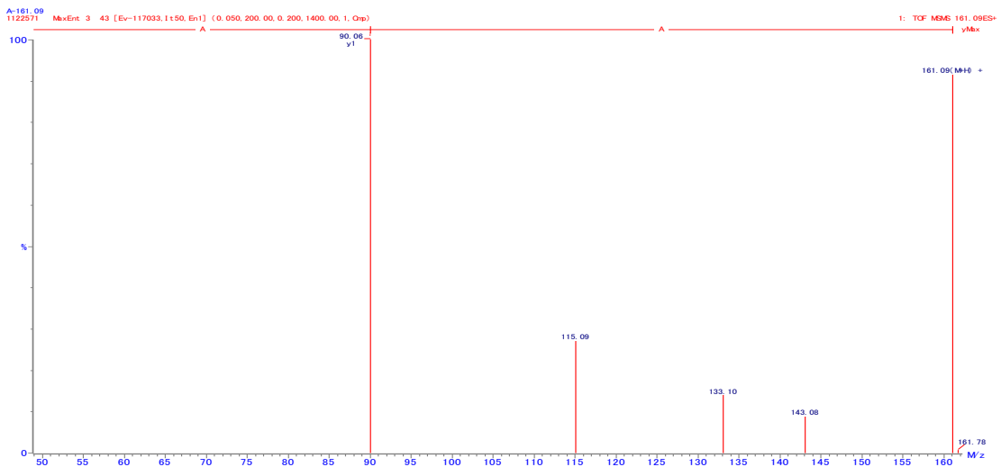
図 15. AA の 2 級質量スペクトル
