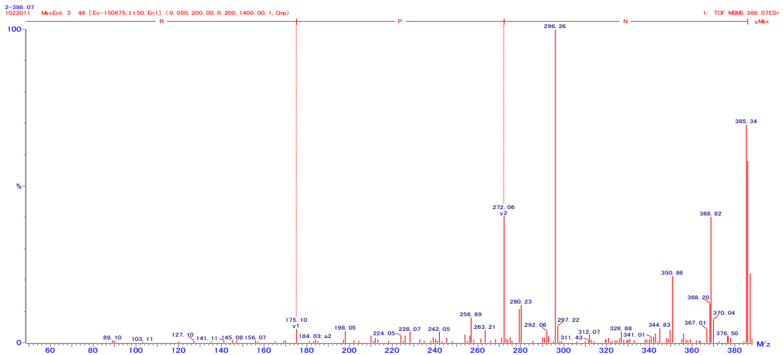
図 9. NPR の 2 級質量スペクトル
