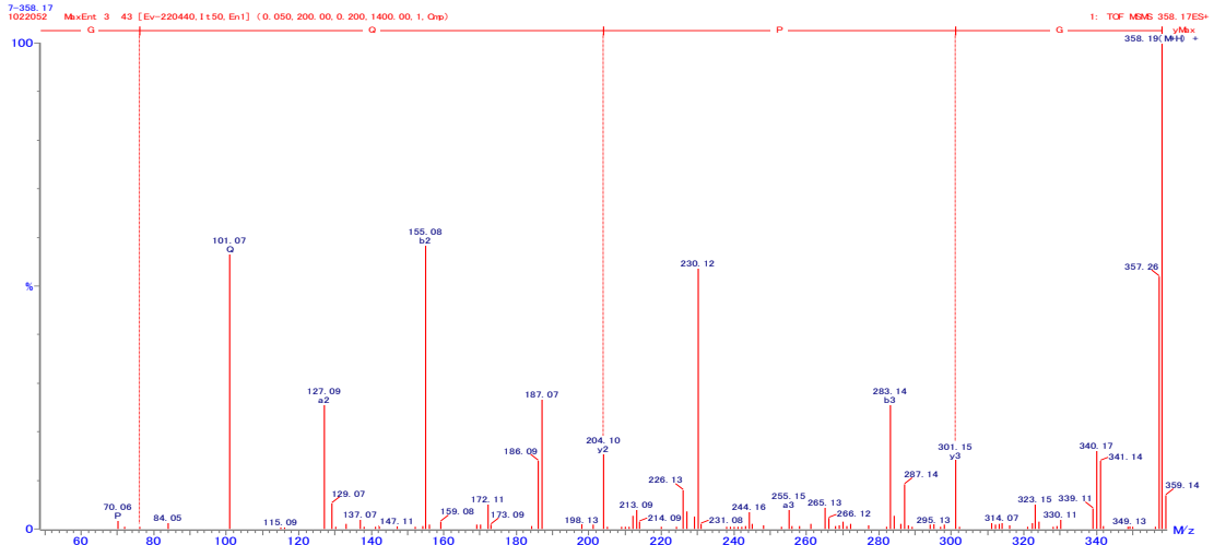
図 31. GPQG の 2 級質量スペクトル
