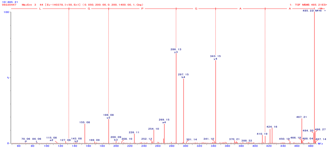
図 46. AAGPGL の 2 級質量スペクトル
