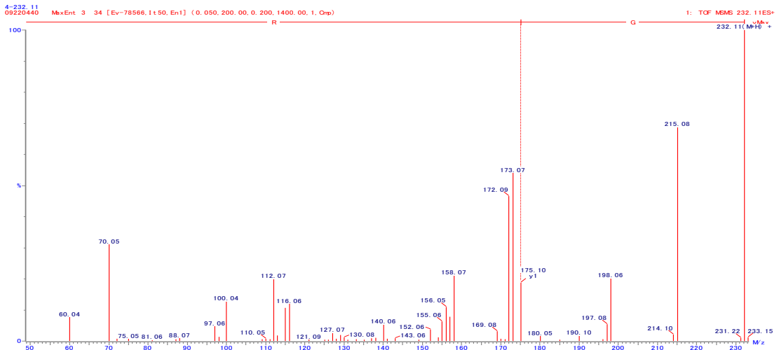
図 18. GR の 2 級質量スペクトル
