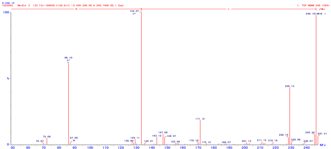
図 36. LN の 2 級質量スペクトル
