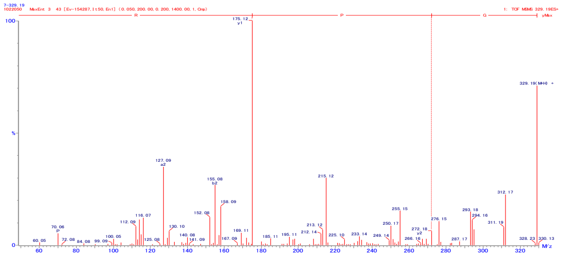
図 30. GPR の 2 級質量スペクトル
