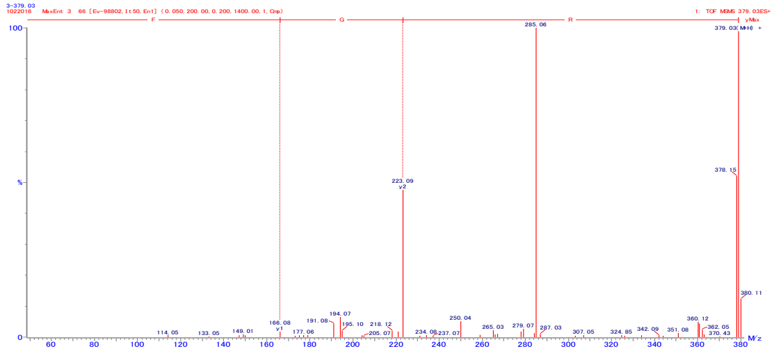
図 11. RGF の 2 級質量スペクトル
