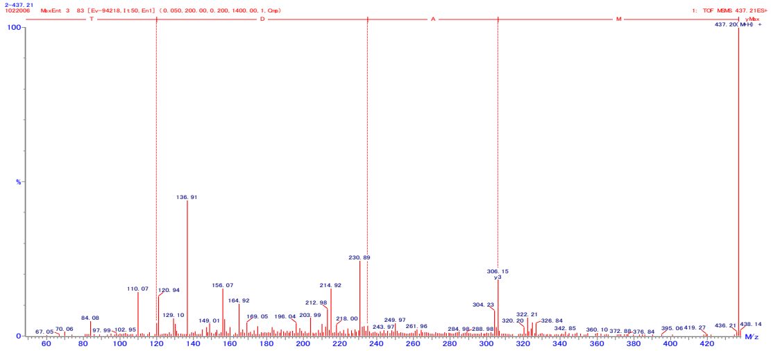
図 7. MADT の 2 級質量スペクトル
