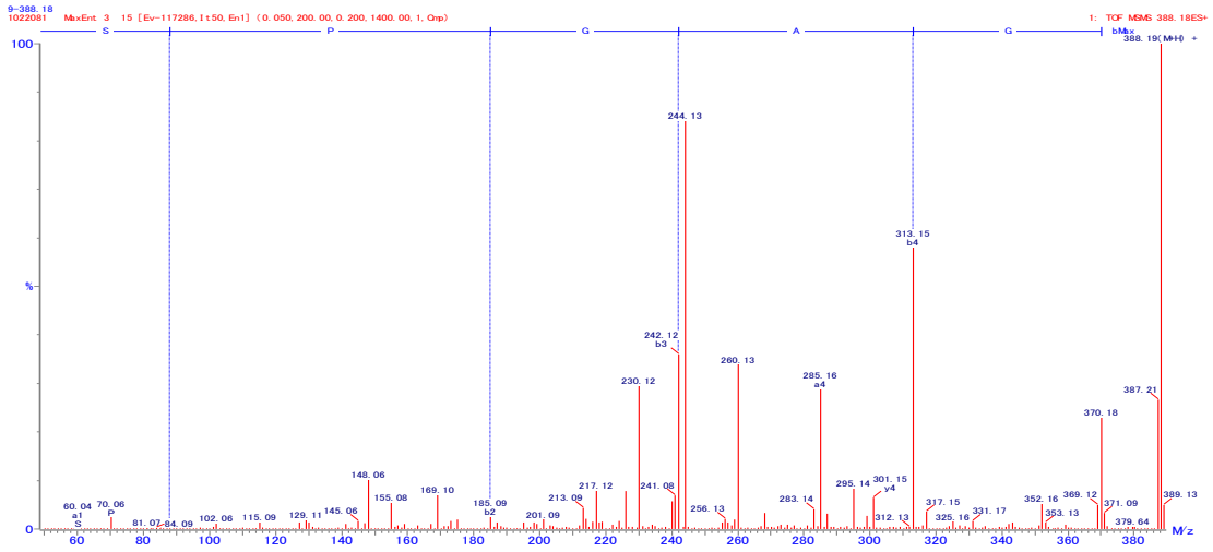
図 41. SPGAG の 2 級質量スペクトル
