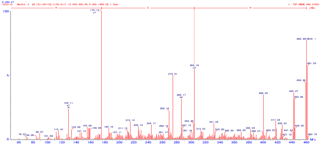
図 28. RER の 2 級質量スペクトル
