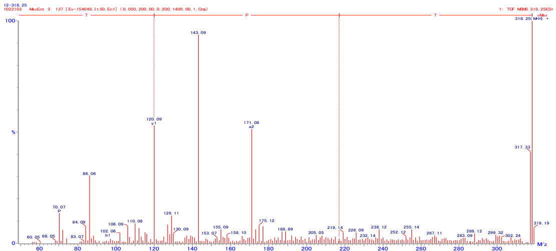
図 57. TPT の 2 級質量スペクトル
