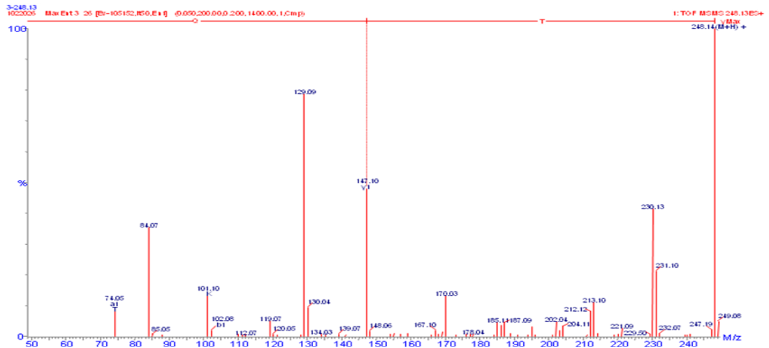
図 10. TQ の 2 級質量スペクトル
