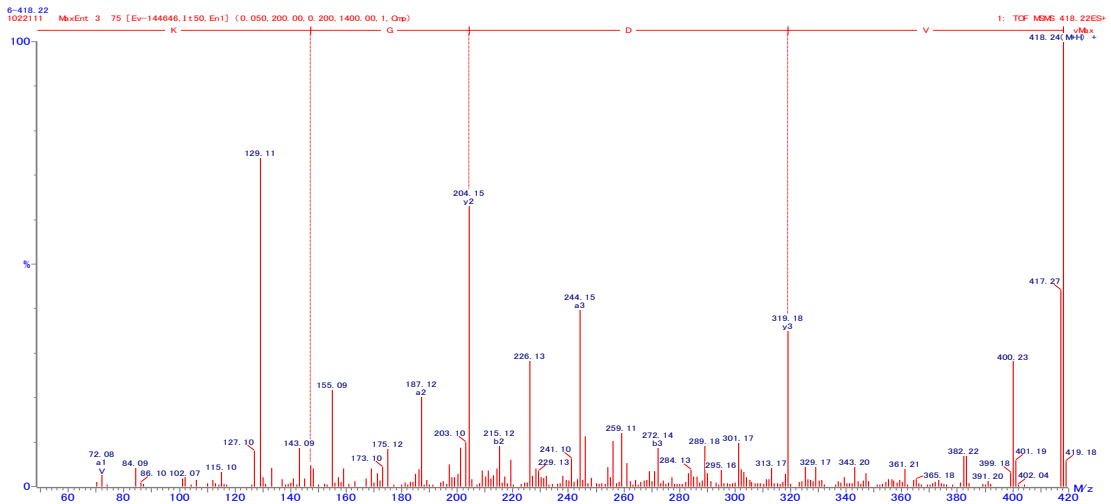
図 27. VDGK の 2 級質量スペクトル
