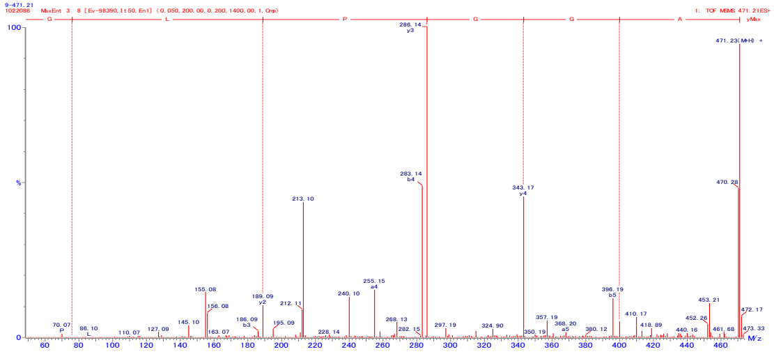
図 43. AGGPLG の 2 級質量スペクトル
