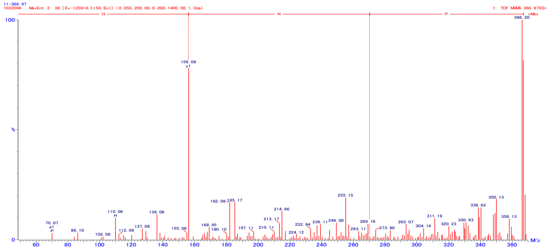
図 53. PNH の 2 級質量スペクトル
