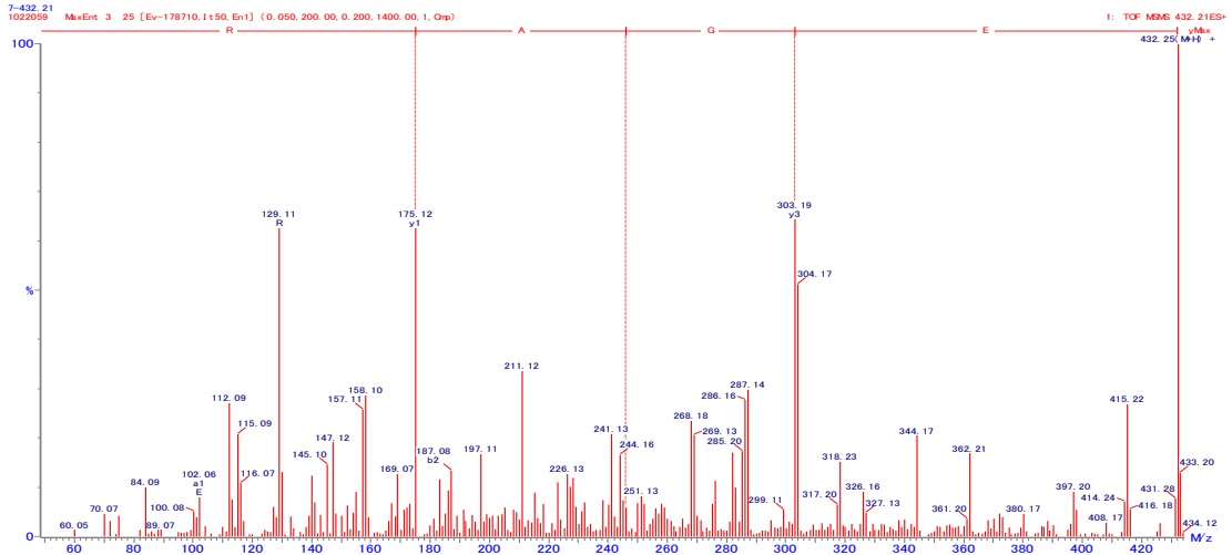
図 34. EGAR の 2 級質量スペクトル
