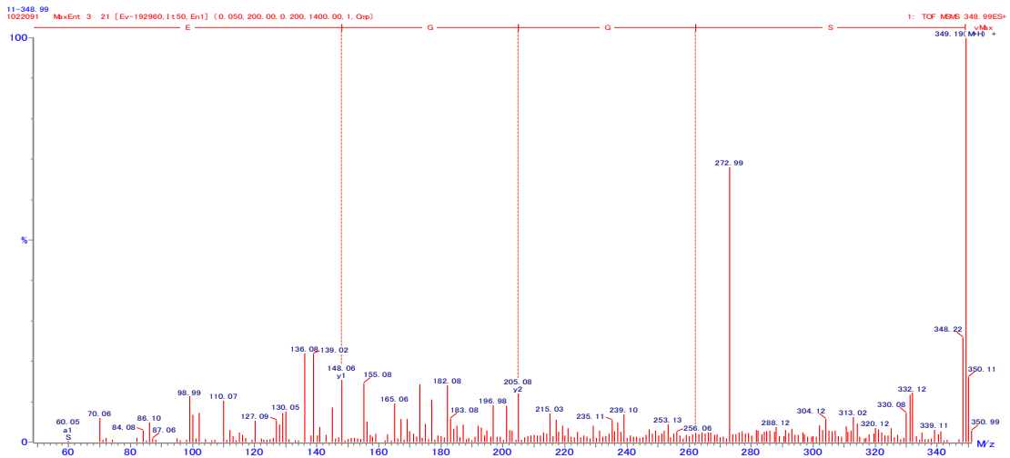
図 50. SGGE の 2 級質量スペクトル
