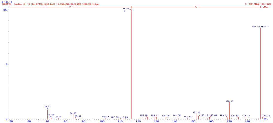
図 26. AP の 2 級質量スペクトル
