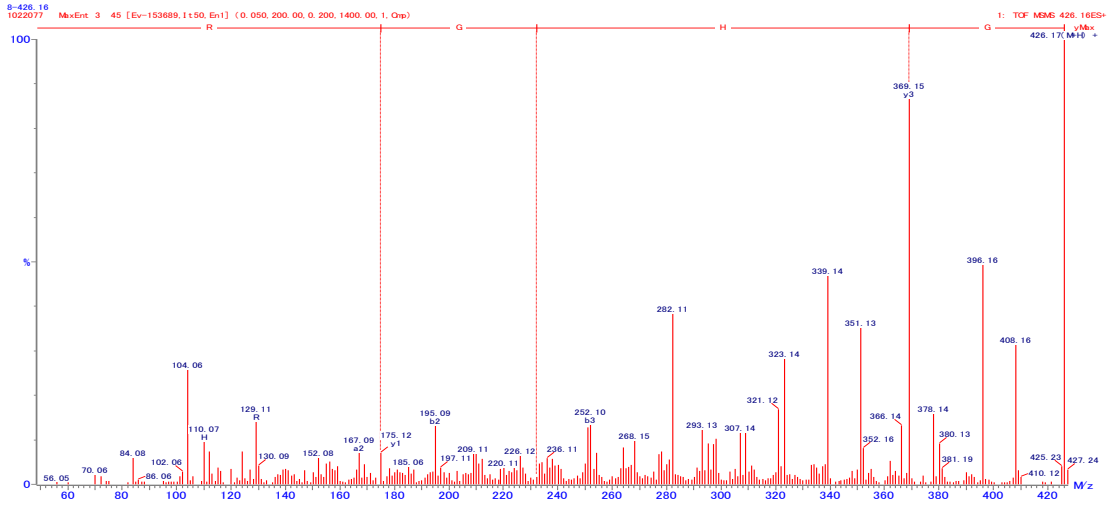
図 40. GHGR の 2 級質量スペクトル
