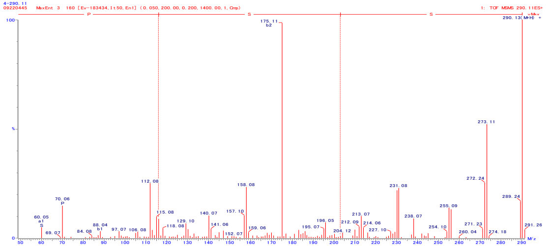
図 19. SSP の 2 級質量スペクトル Fig.19 The MS/MS spectrum of SSP
