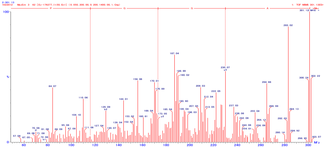
図 5. AGGP の 2 級質量スペクトル
