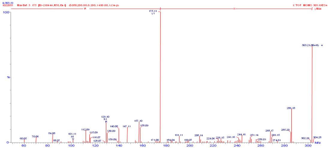
図 20. KR の 2 級質量スペクトル Fig.20 The MS/MS spectrum of KR
