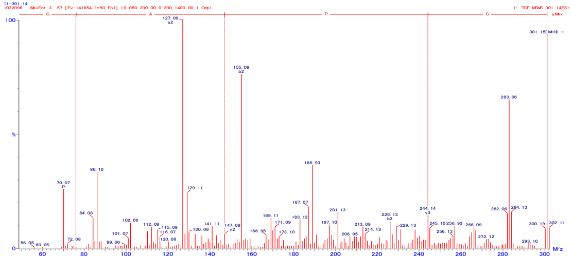
図 52. GPAG の 2 級質量スペクトル
