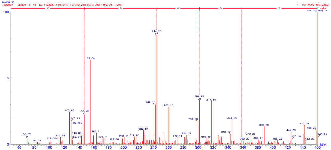
図 44. TGGPK の 2 級質量スペクトル
