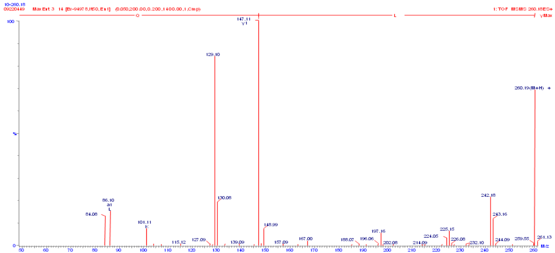
図 49. LQ の 2 級質量スペクトル
