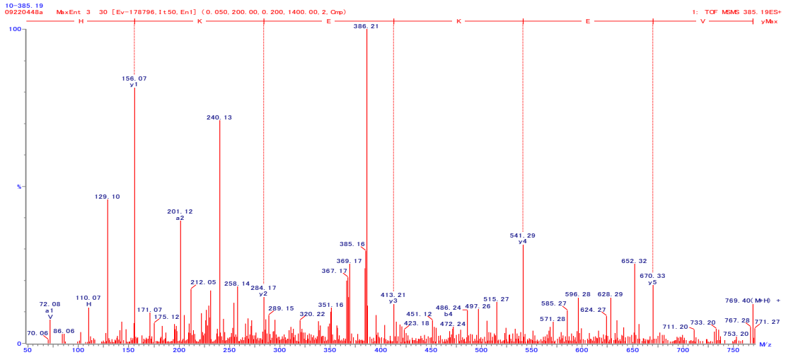
図 47. VEKEKH の 2 級質量スペクトル
