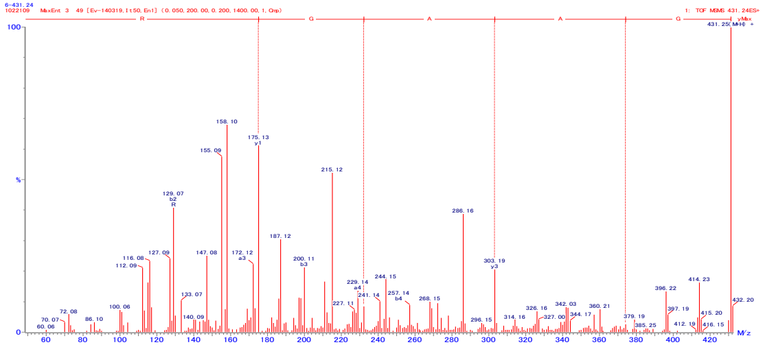
図 25. GAAGR の 2 級質量スペクトル
