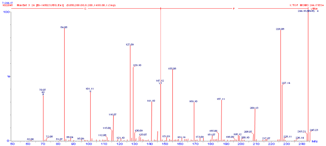
図 29. PQ の 2 級質量スペクトル
