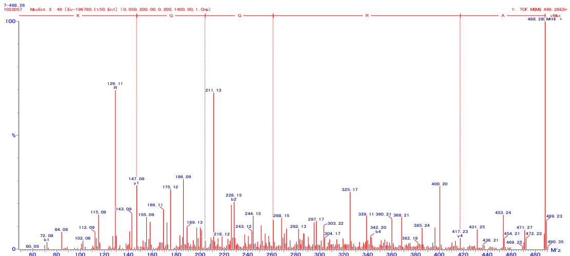
図 33. ARGGK の 2 級質量スペクトル
