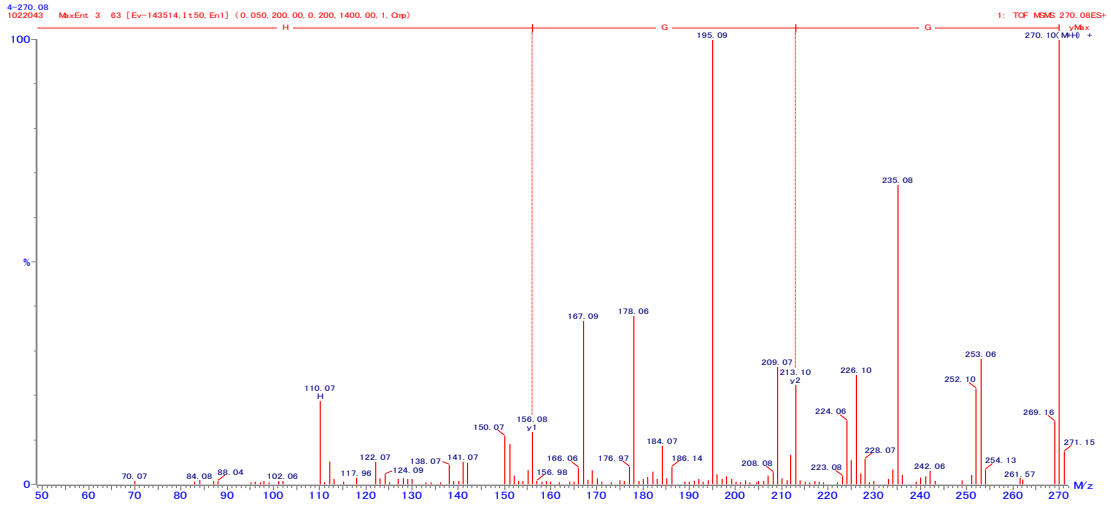
図 22. GGH の 2 級質量スペクトル
