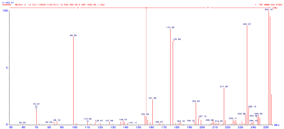
図 54. PH の 2 級質量スペクトル
