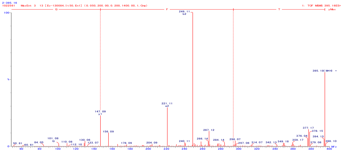
図 12. TFQ の 2 級質量スペクトル
