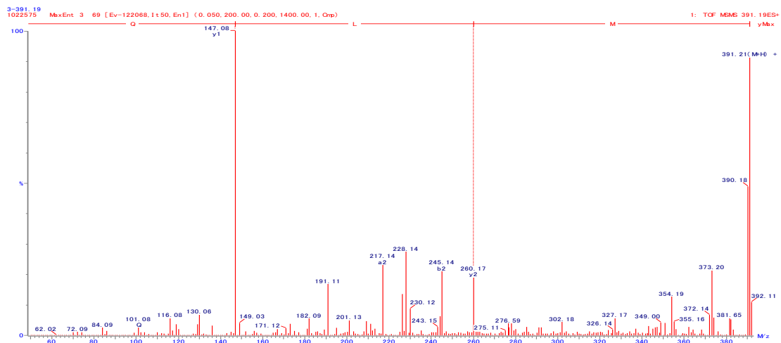
図 17. MLQ の 2 級質量スペクトル
