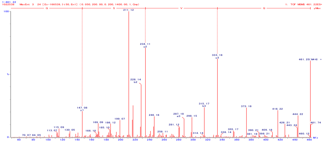
図 1. QVSQ の 2 級質量スペクトル
