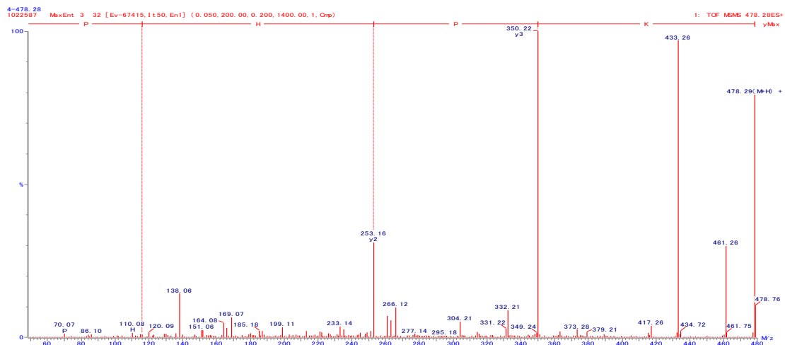
図 20. KPHP の 2 級質量スペクトル
