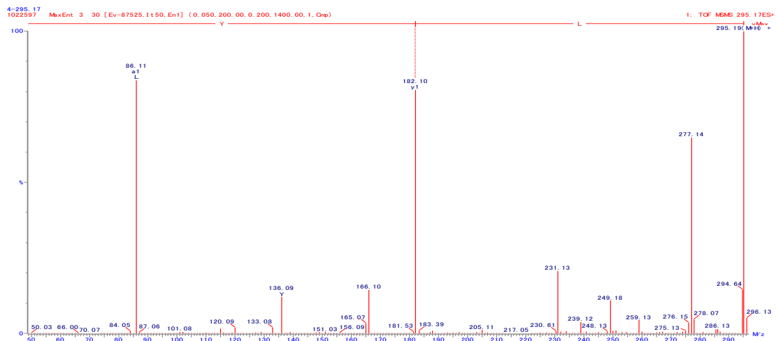
図 26. LY の 2 級質量スペクトル
