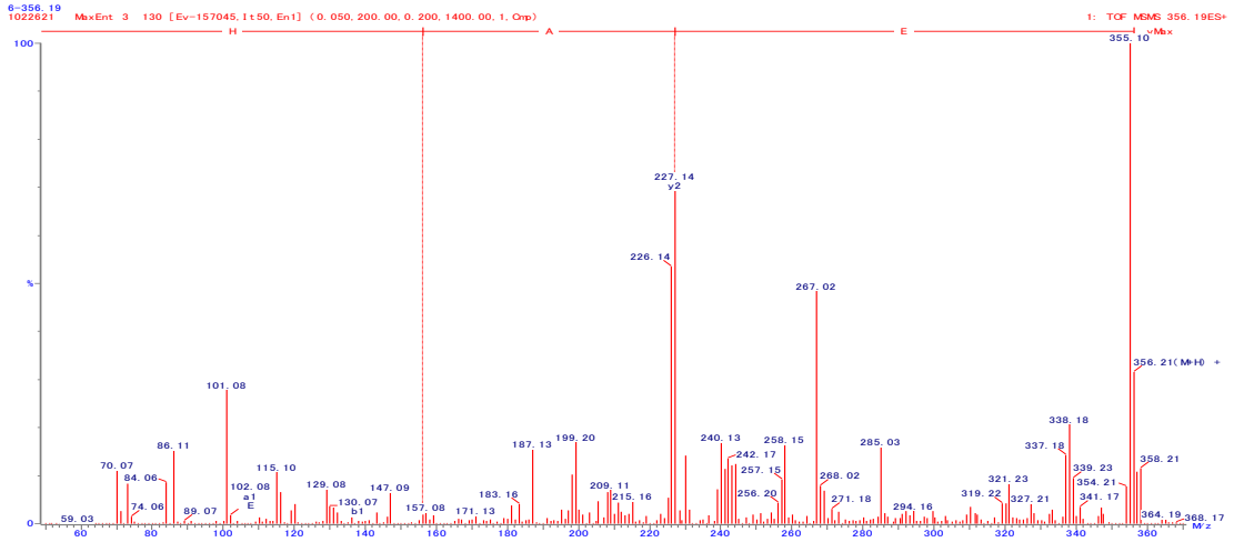
図 37. EAH の 2 級質量スペクトル
