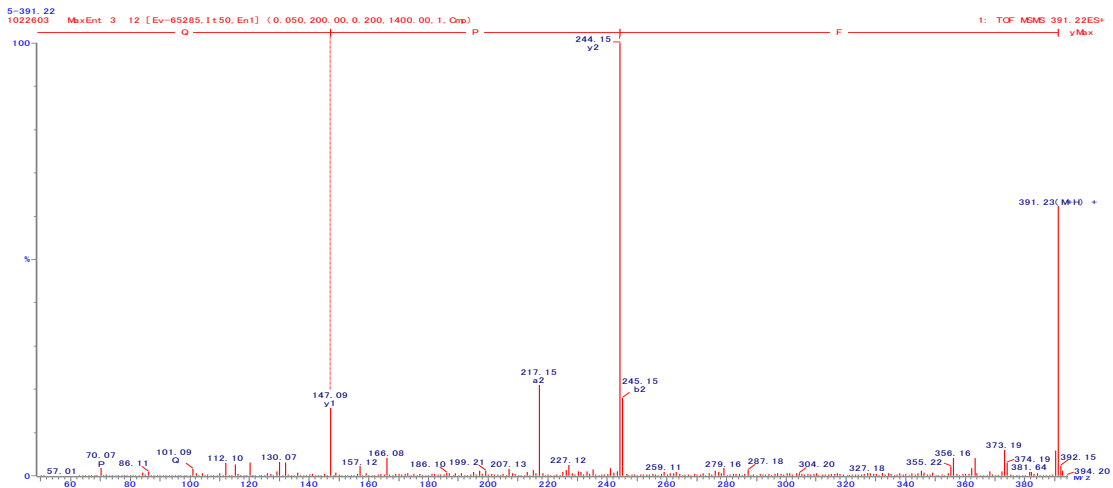
図 30. FPQ の 2 級質量スペクトル
