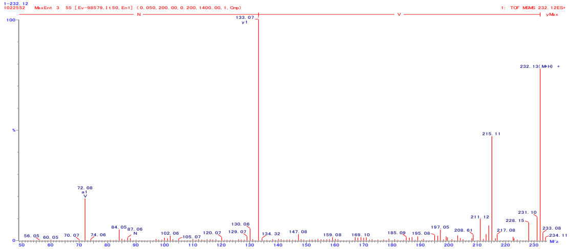
図7. VNの2級質量スペクトル
