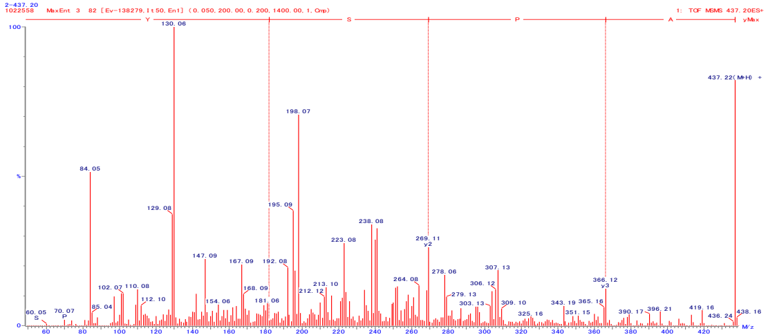
図 10. APSY の 2 級質量スペクトル
