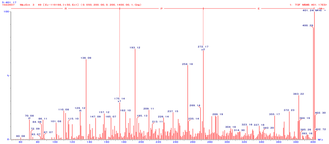
図 32. EPR の 2 級質量スペクトル
