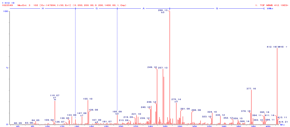
図 5. HGAQ の 2 級質量スペクトル
