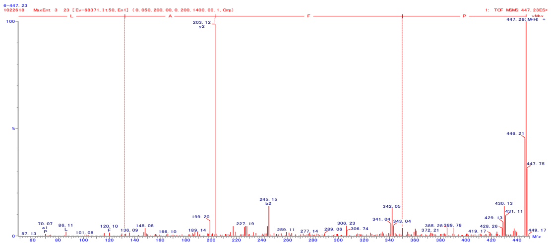
図 36. PFAL の 2 級質量スペクトル
