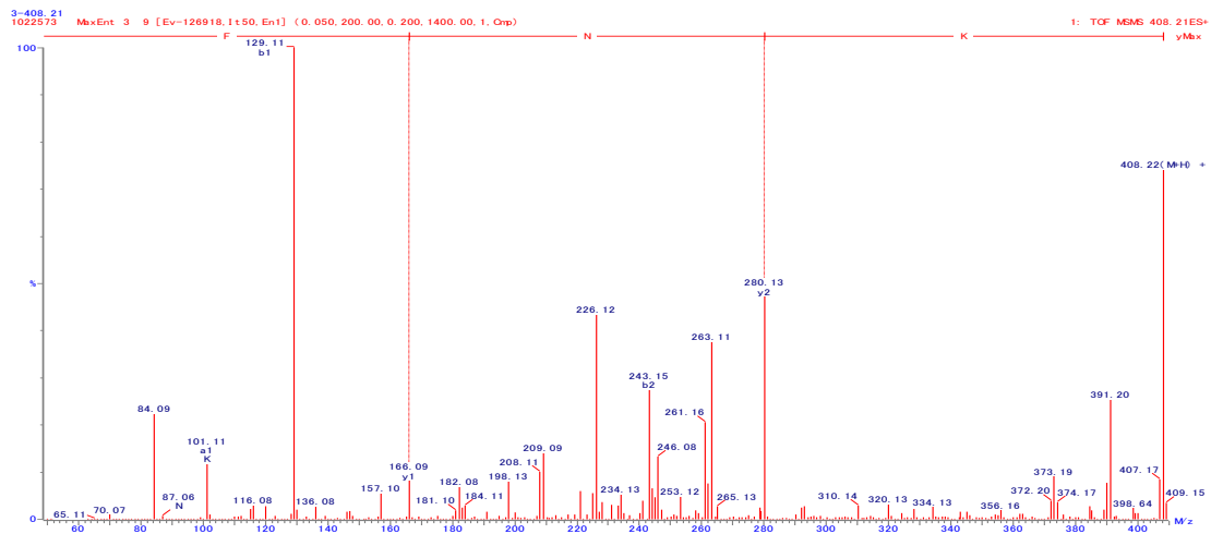
図 16. KNF の 2 級質量スペクトル
