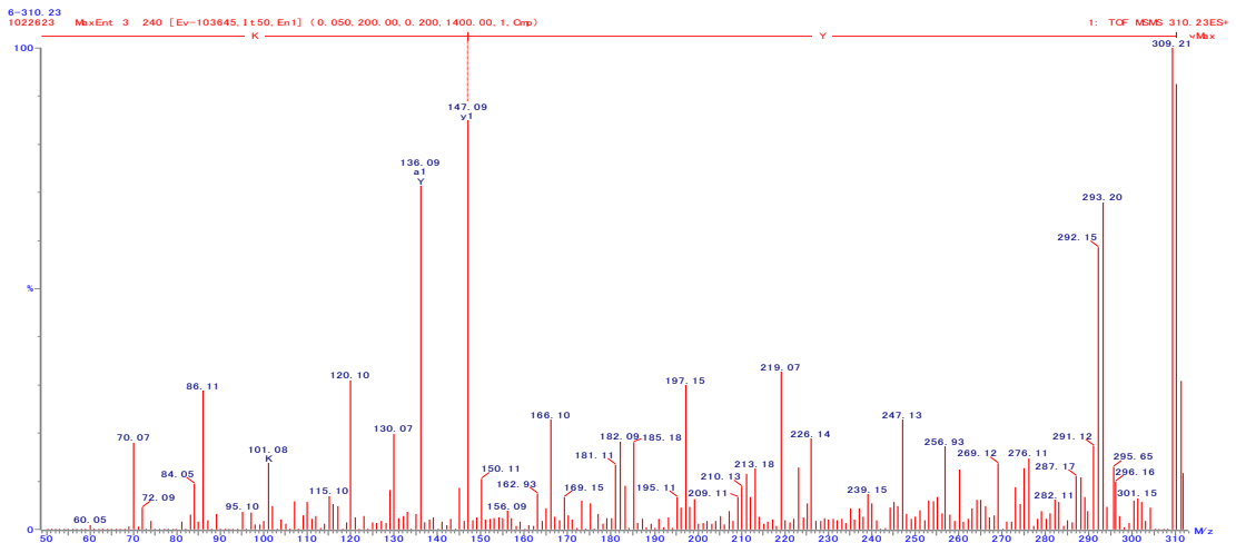
図 39. YQ の 2 級質量スペクトル
