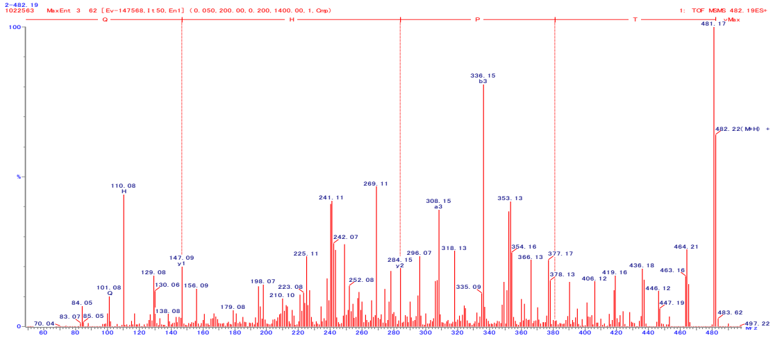
図 13. TPHQ の 2 級質量スペクトル Fig.13 The MS/MS spectrum of TPHQ
