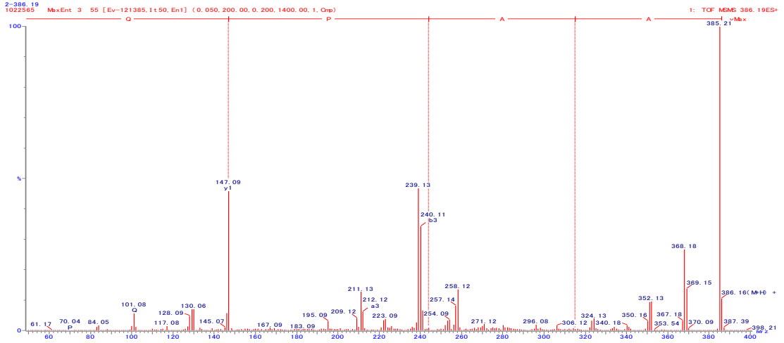
図 14. AAPQ の 2 級質量スペクトル Fig.14 The MS/MS spectrum of AAPQ
