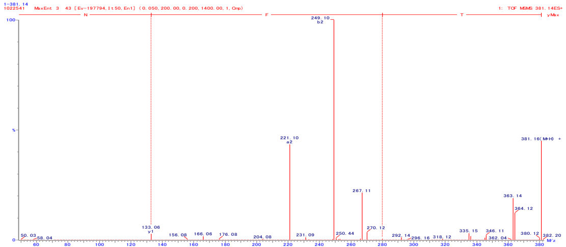
図 2. TFN の 2 級質量スペクトル
