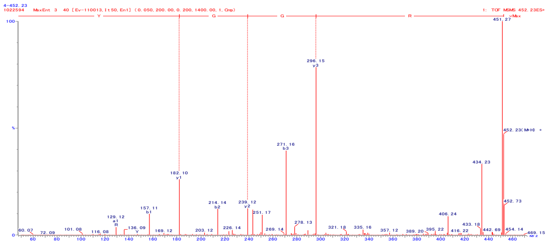
図 24. RGGY の 2 級質量スペクトル
