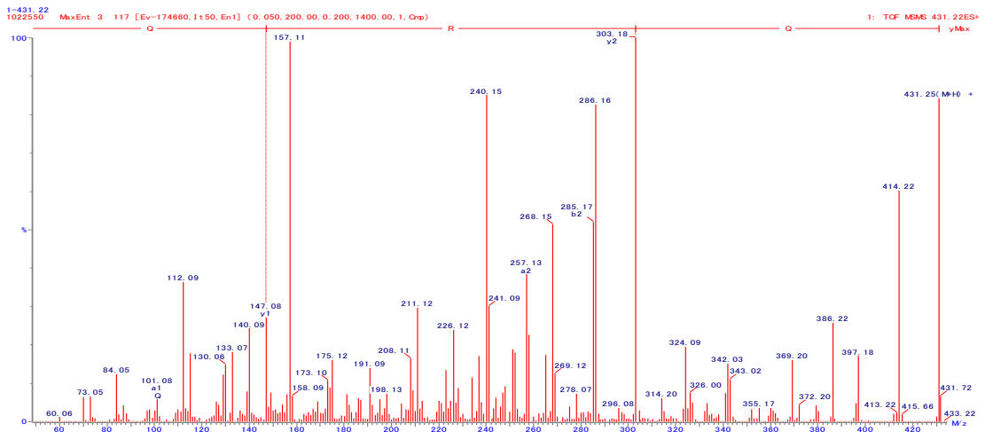
図 6. QRQ の 2 級質量スペクトル
