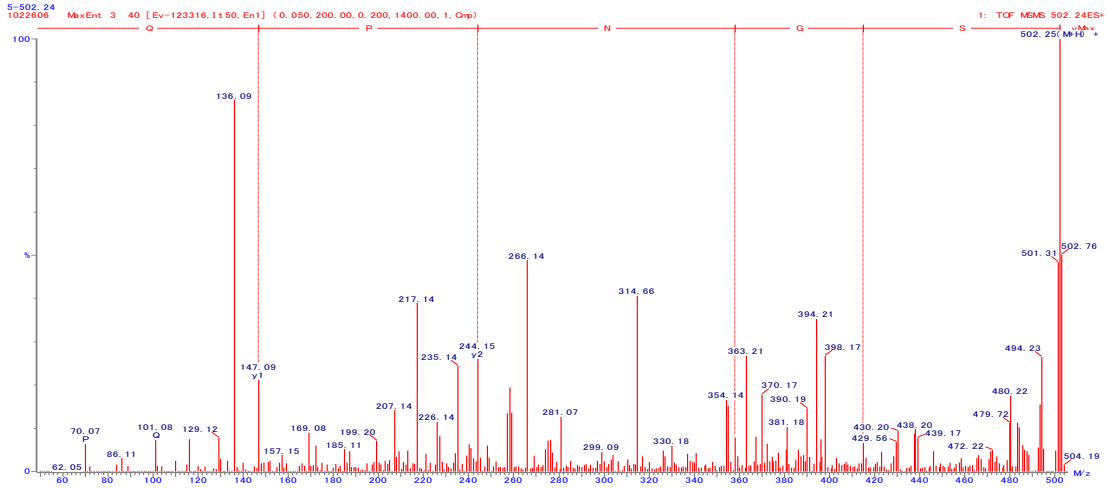
図 31. SGNPQ の 2 級質量スペクトル
