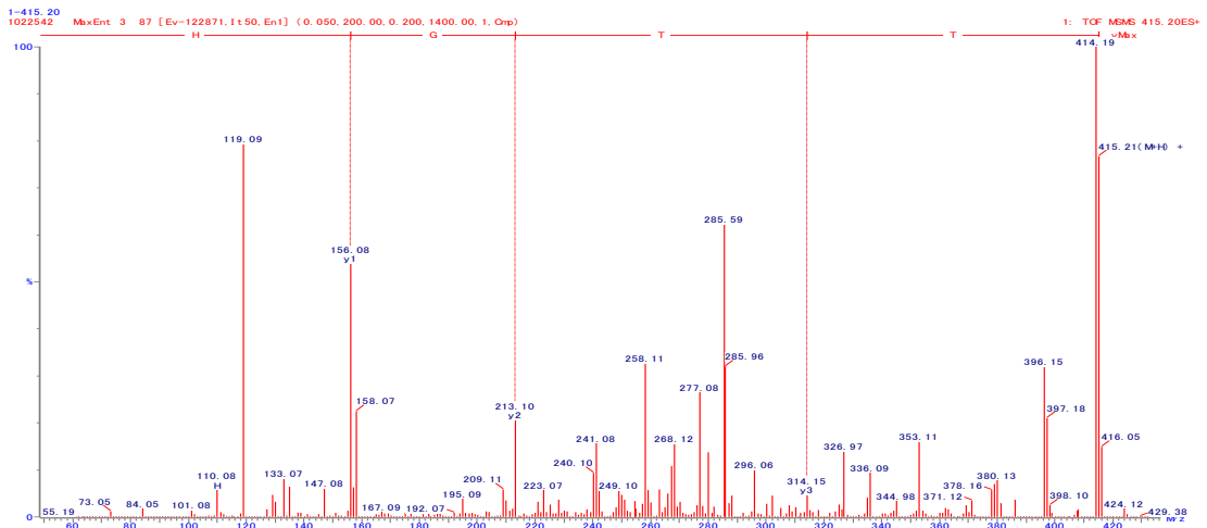
図 3. TTGH の 2 級質量スペクトル
