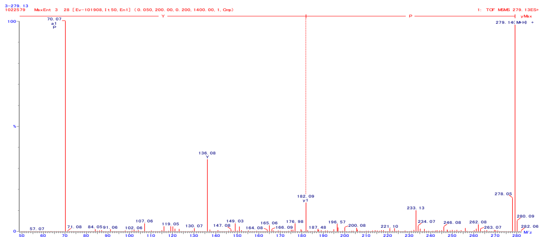
図 19. PY の 2 級質量スペクトル
