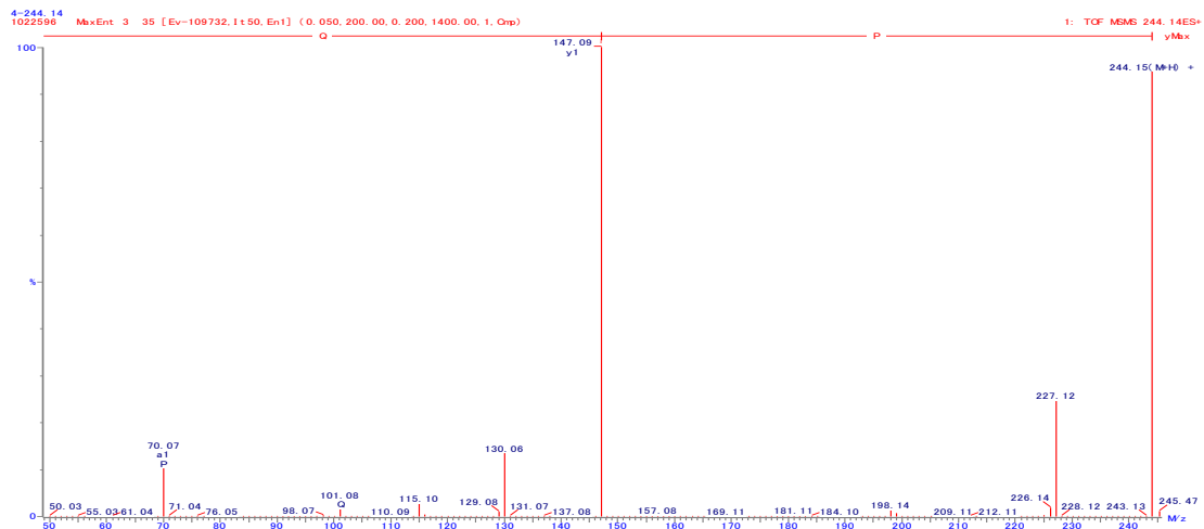
図 25. PQ の 2 級質量スペクトル
