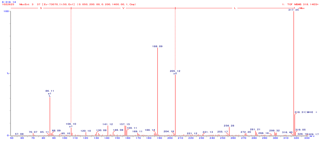
図 40. LVS の 2 級質量スペクトル
