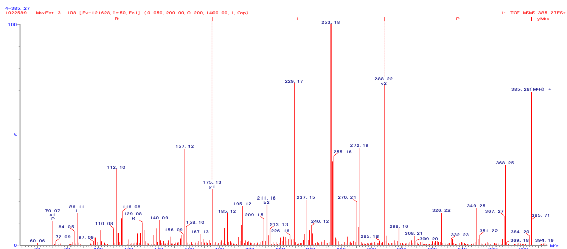
図 21. PLR の 2 級質量スペクトル
