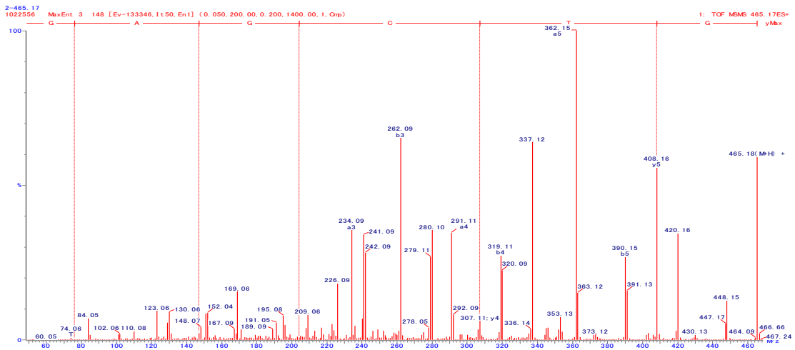
図9. GTCGAGの2級質量スペクトル
