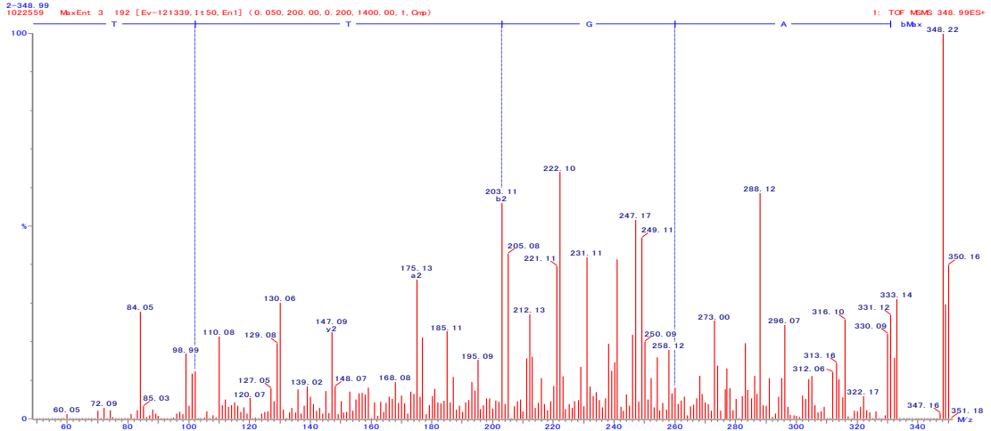
図 11. TTGA の 2 級質量スペクトル
