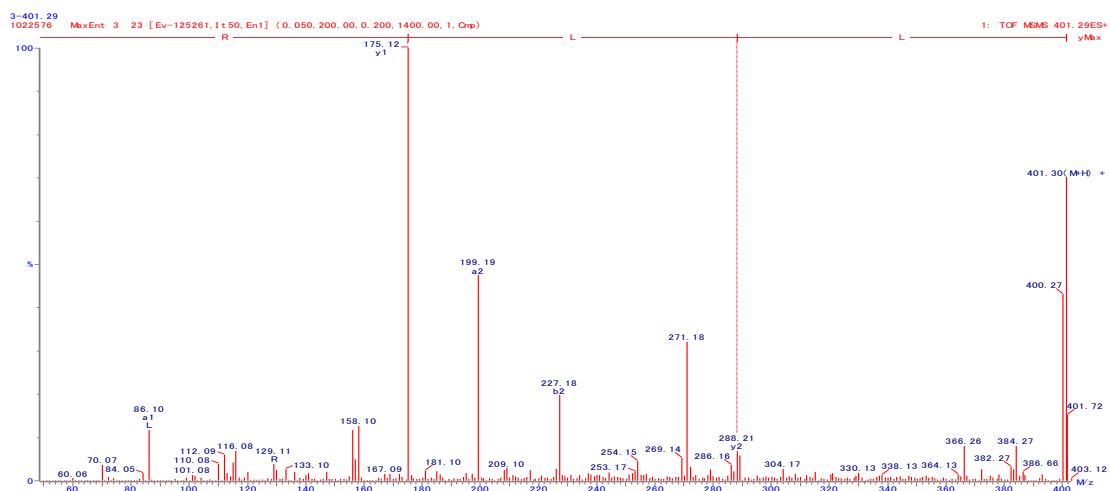
図 18. ILR の 2 級質量スペクトル
