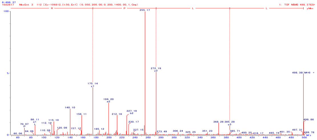
図 35. ILPR の 2 級質量スペクトル
