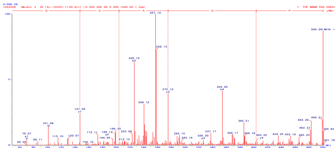
図 27. PQAGQ の 2 級質量スペクトル
