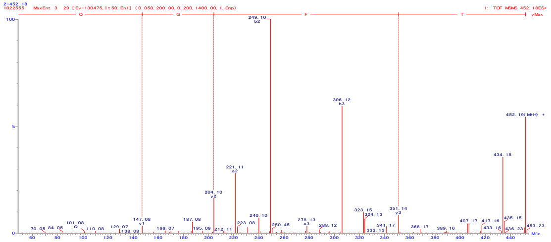
図8. TFGQの2級質量スペクトル
