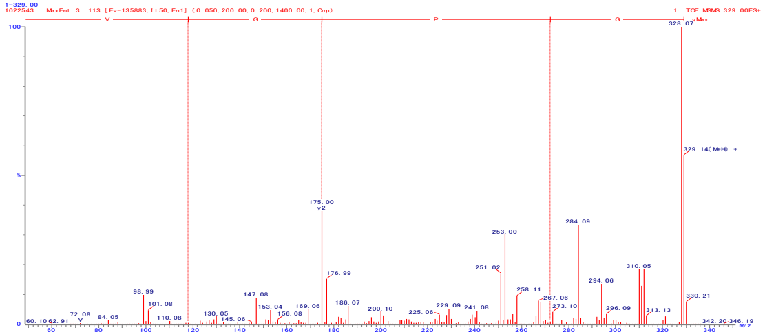
図 4. GPGV の 2 級質量スペクトル
