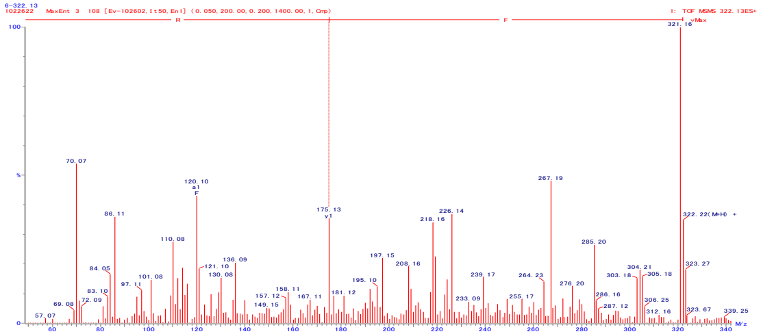
図 38. FR の 2 級質量スペクトル
