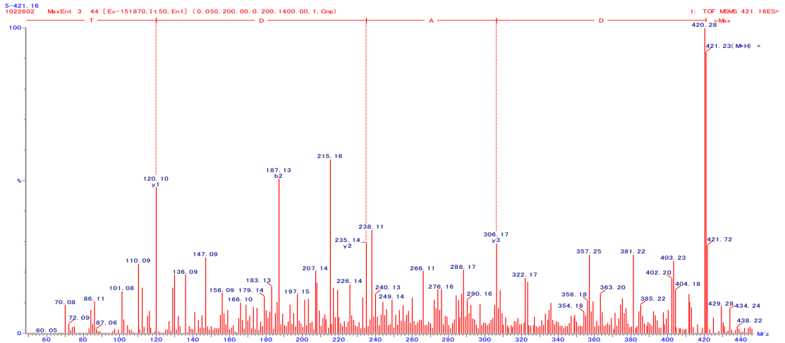
図 29. DADT の 2 級質量スペクトル
