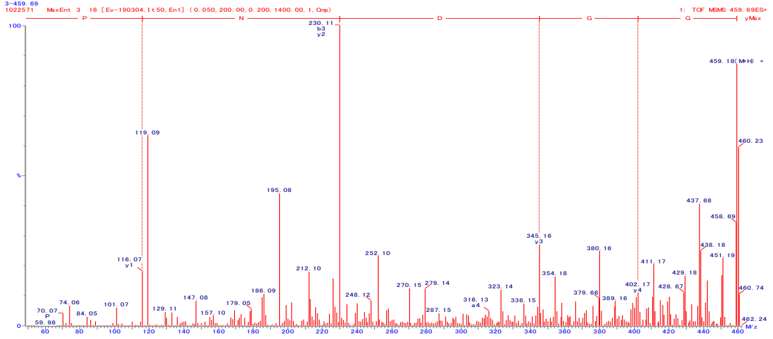
図 15. GGDNP の 2 級質量スペクトル Fig.15 The MS/MS spectrum of GGDNP
