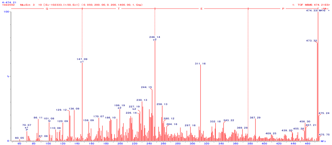
図 23. PETQ の 2 級質量スペクトル
