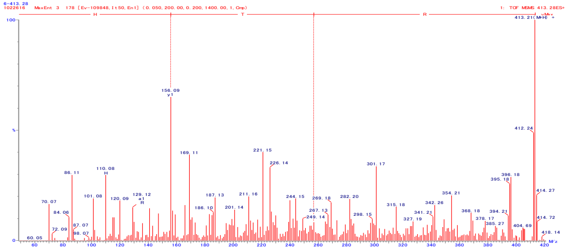
図 34. RTH の 2 級質量スペクトル
