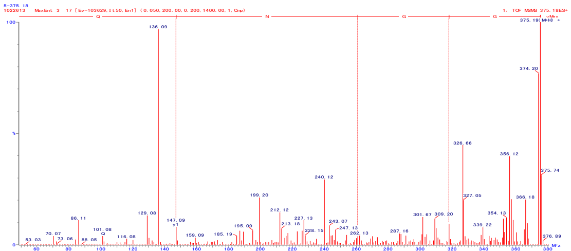
図 33. GGNQ の 2 級質量スペクトル
