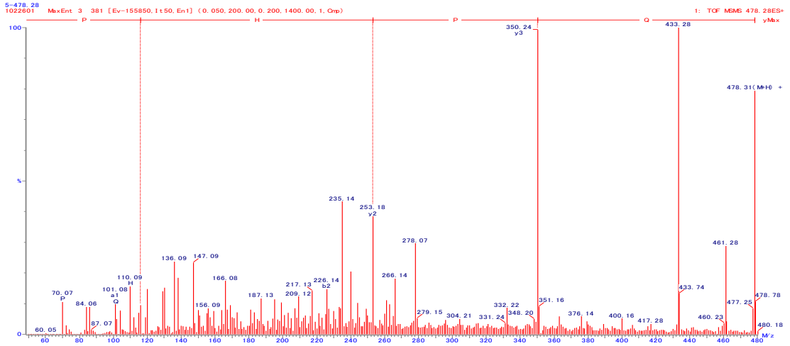
図 28. QPHP の 2 級質量スペクトル
