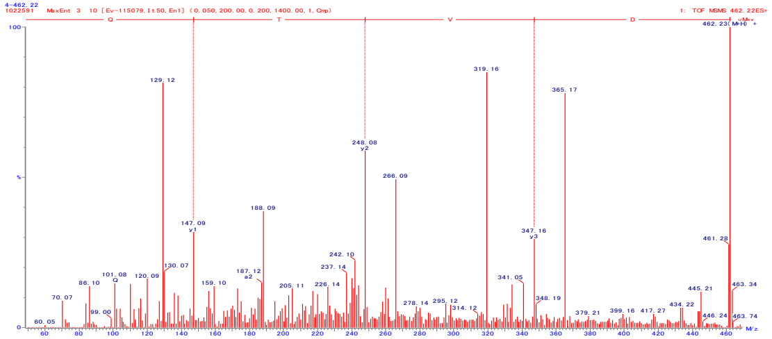
図 22. DVTQ の 2 級質量スペクトル
