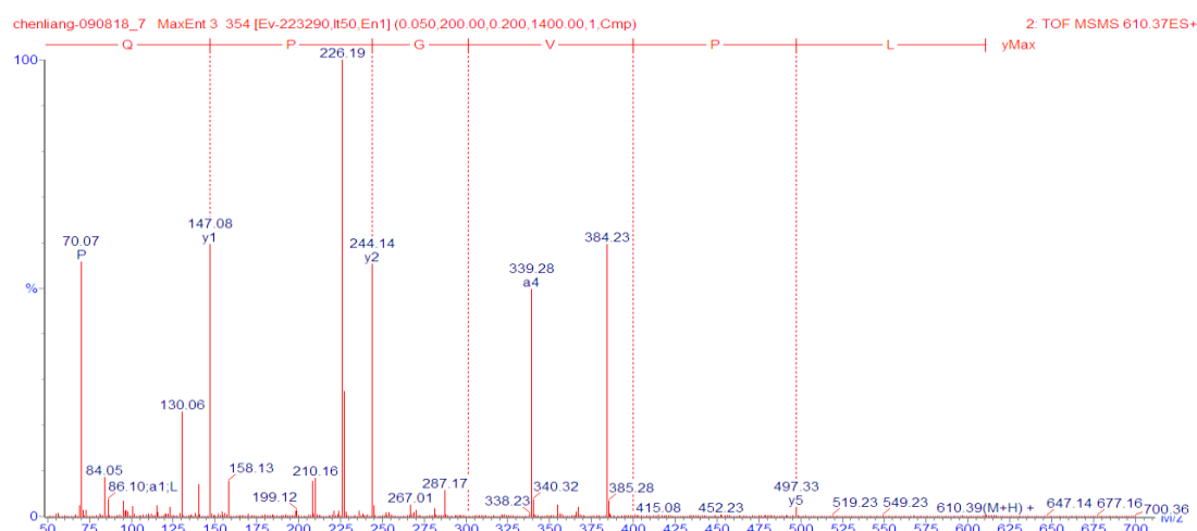
図 33. LPVGPQ の 2 級質量スペクトル
