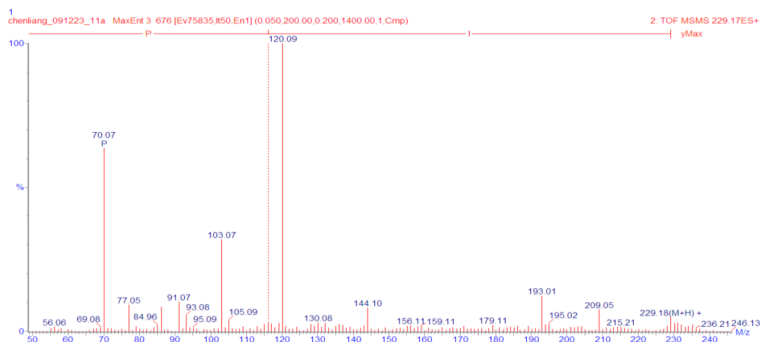
図 50. IP の 2 級質量スペクトル
