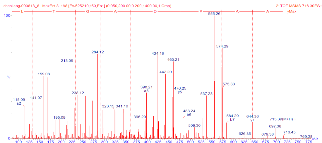
図 42. AAPDAGTL の 2 級質量スペクトル
