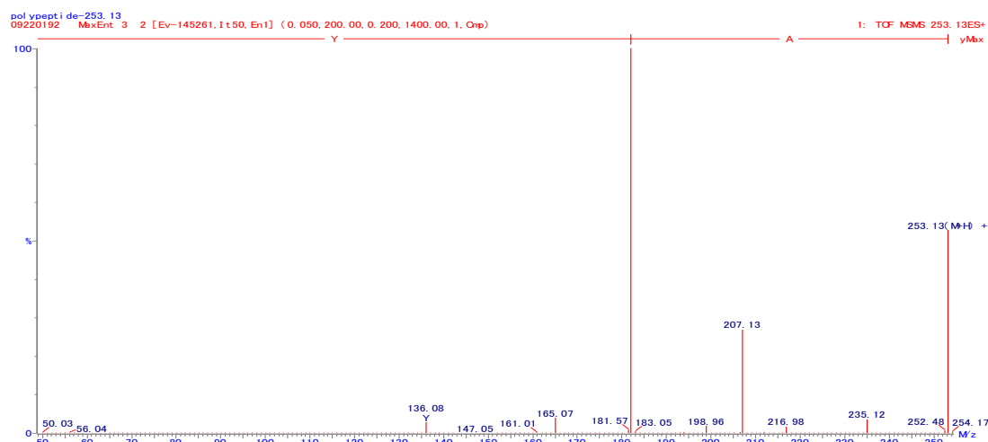
図 11. AY の 2 級質量スペクトル
