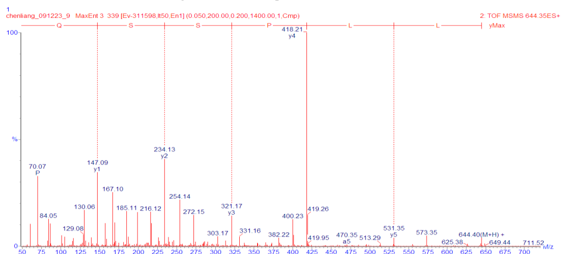
図 36. LLPSSQ の 2 級質量スペクトル
