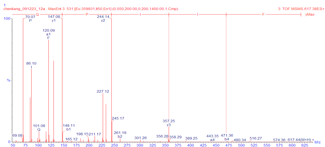
図 56. FIIPQ の 2 級質量スペクトル
