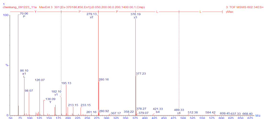
図 53. LLPPY の 2 級質量スペクトル
