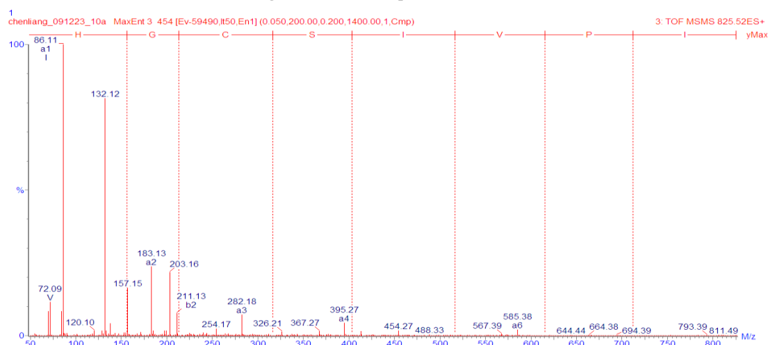
図 48. IPVISCGH の 2 級質量スペクトル
