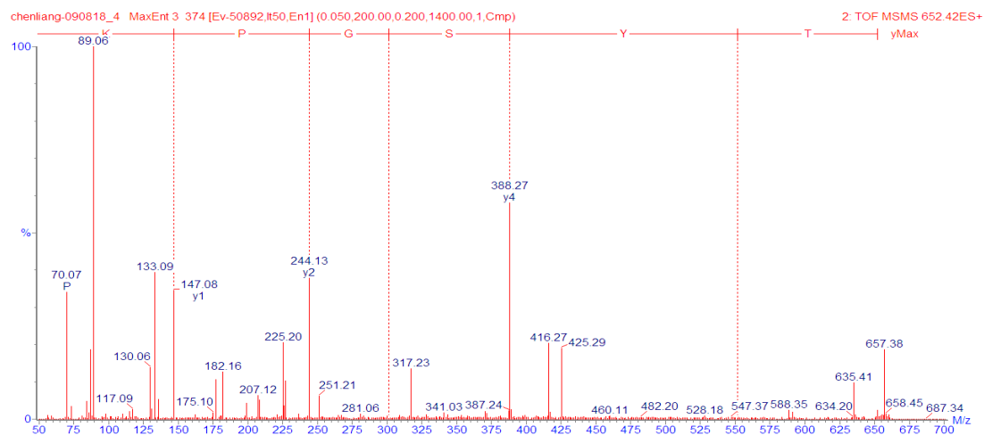
図 17. TYSGPK の 2 級質量スペクトル
