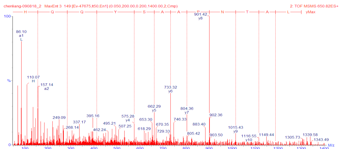
図 9. LATNPAASYQQH の 2 級質量スペクトル
