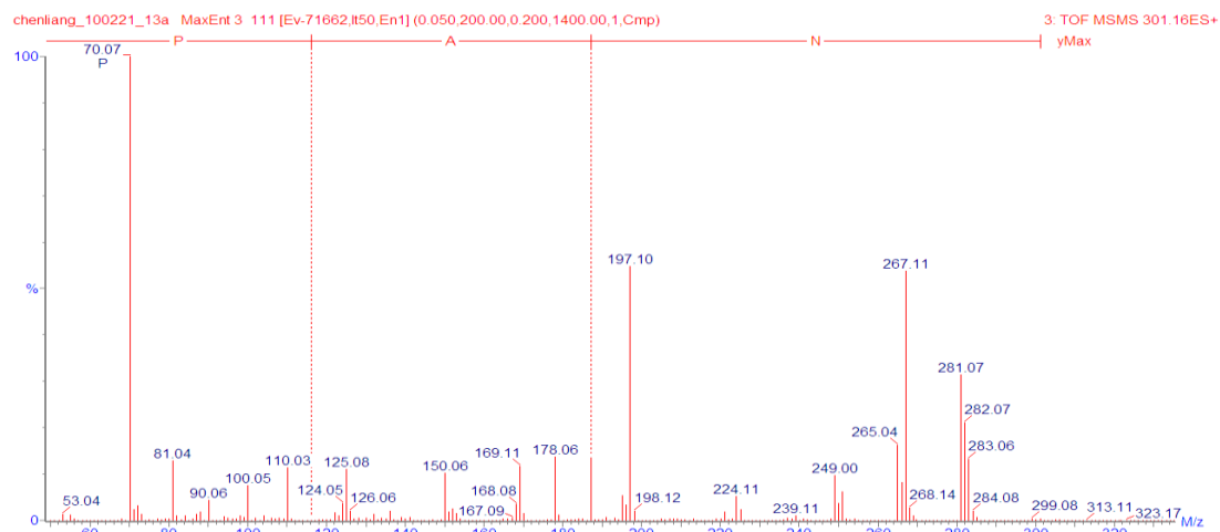
図 13. NAP の 2 級質量スペクトル
