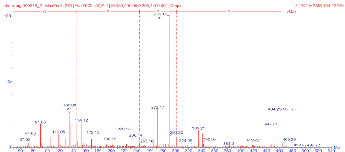
図 7. YGPQ の 2 級質量スペクトル
