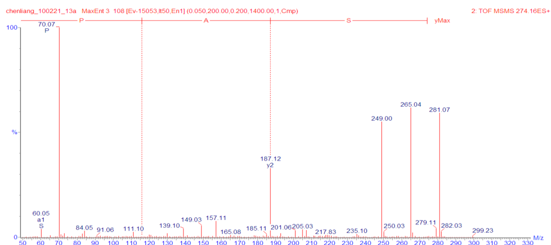
図 12. SAP の 2 級質量スペクトル
