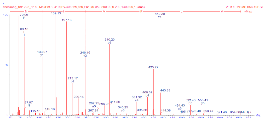
図 49. VLPVIN の 2 級質量スペクトル
