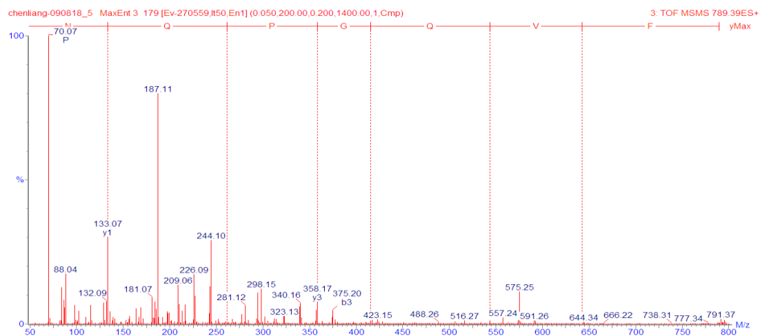
図 21. FVQGPQN の 2 級質量スペクトル
