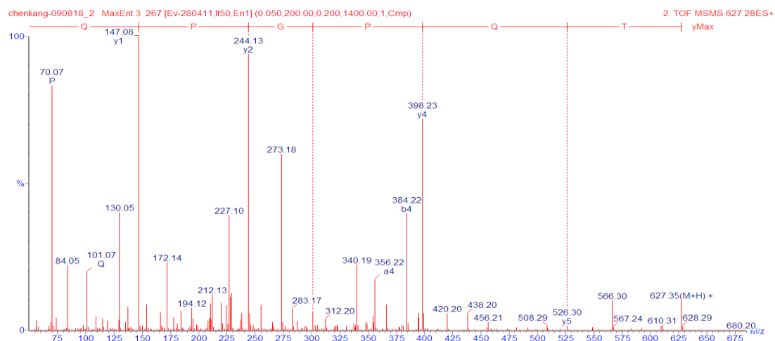
図 8. TQPGPQ の 2 級質量スペクトル
