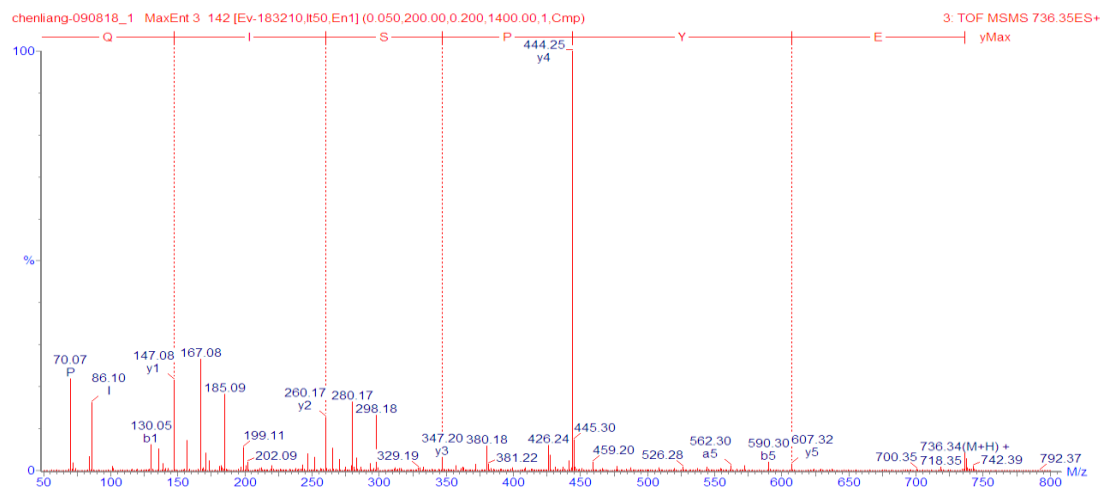
図 4. EYPSIQ の 2 級質量スペクトル
