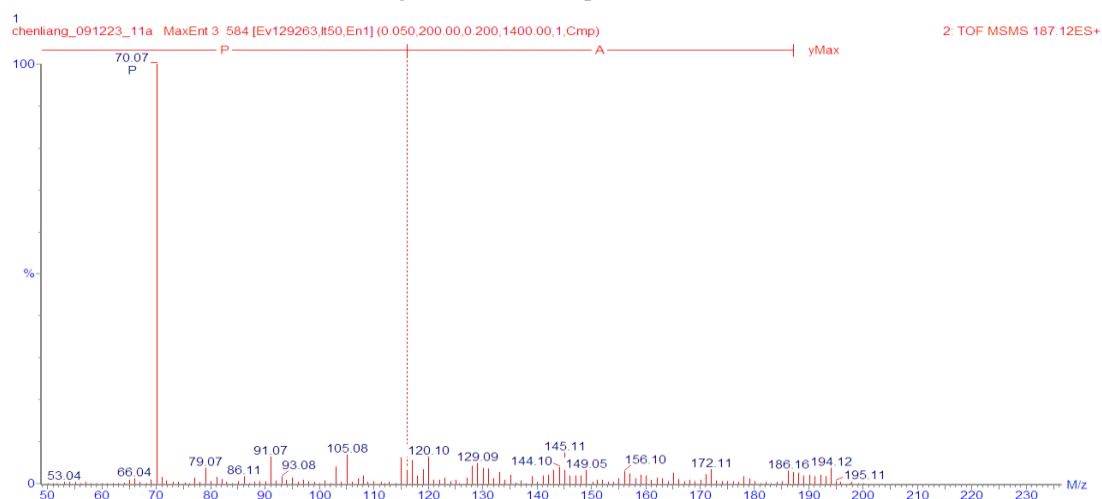
図 51. AP の 2 級質量スペクトル
