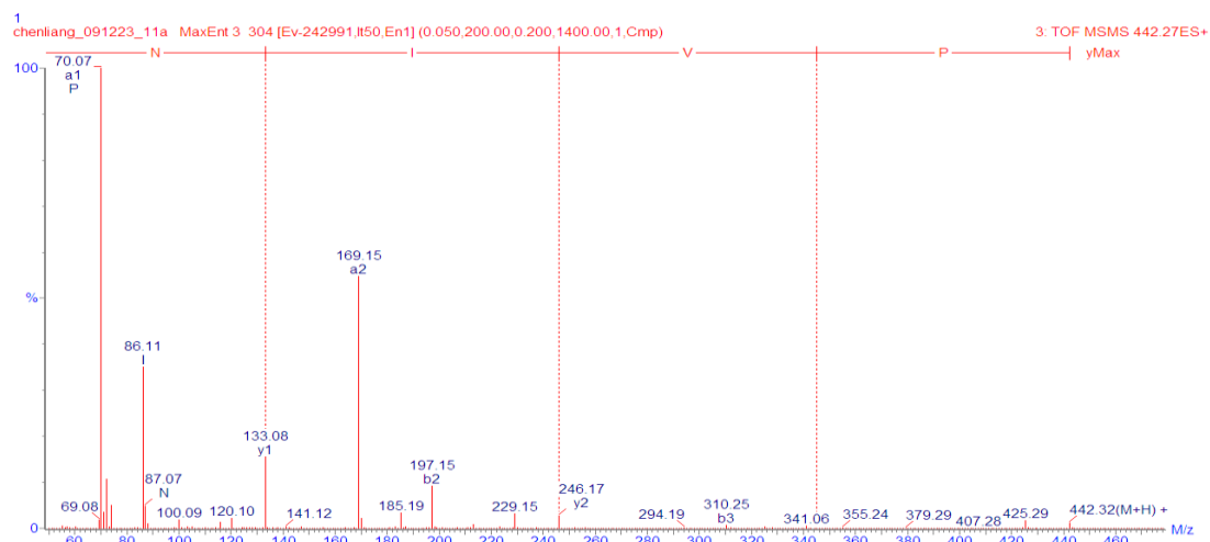
図 52. PVIN の 2 級質量スペクトル
