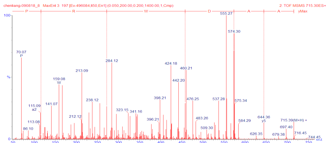
図 32. AADWRP の 2 級質量スペクトル
