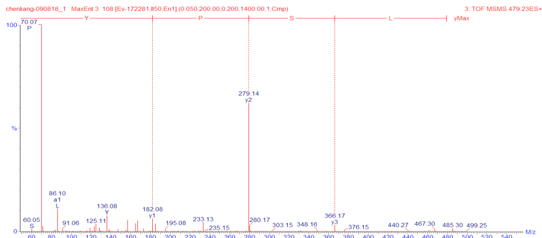
図 1. LSPY の 2 級質量スペクトル
