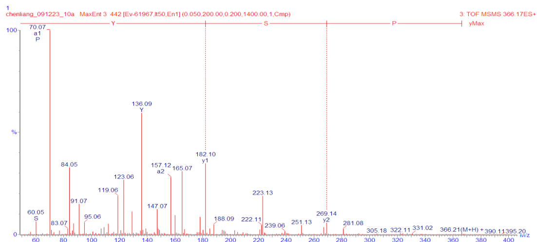
図 46. PSY の 2 級質量スペクトル
