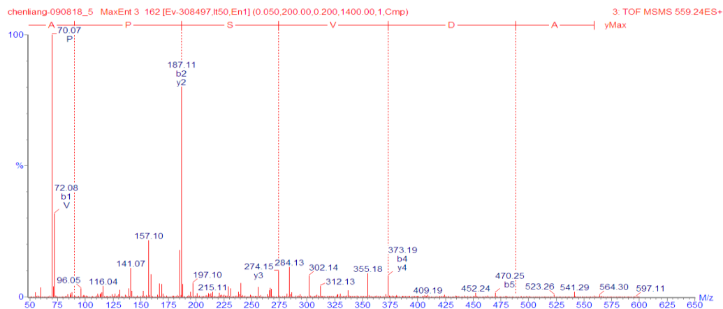
図 19. ADVSPA の 2 級質量スペクトル
