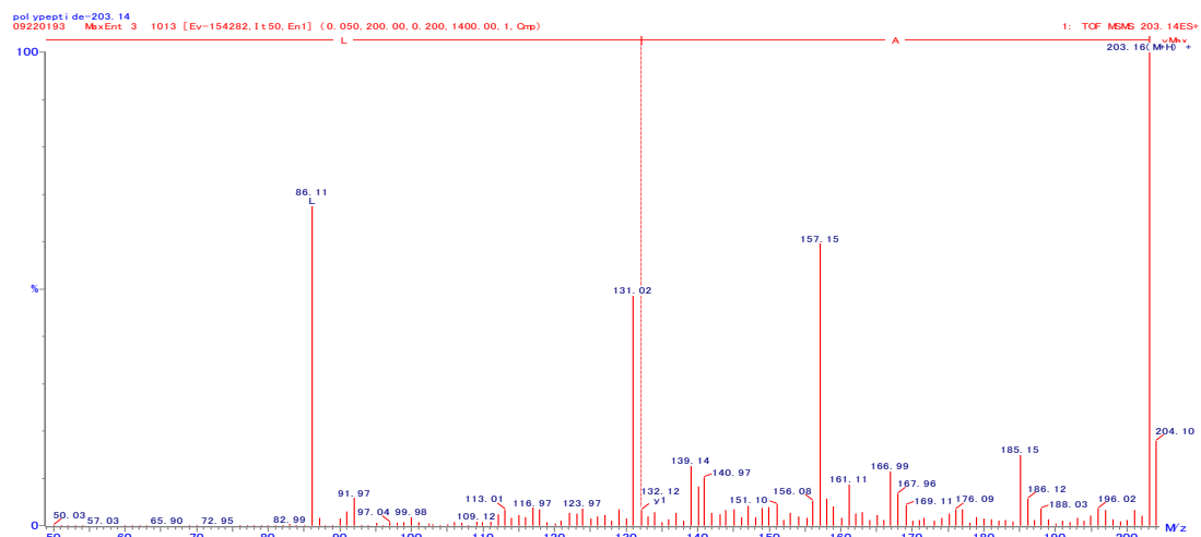
図 10. AL の 2 級質量スペクトル
