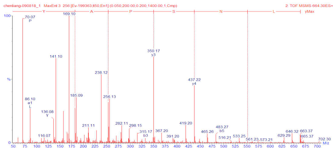
図 2. LNSPAY の 2 級質量スペクトル
