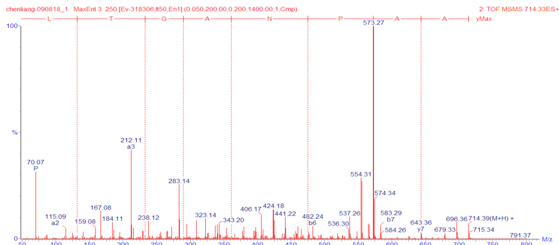
図 3. AAPNAGTL の 2 級質量スペクトル
