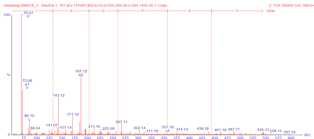
図 23. VSPGAL の 2 級質量スペクトル
