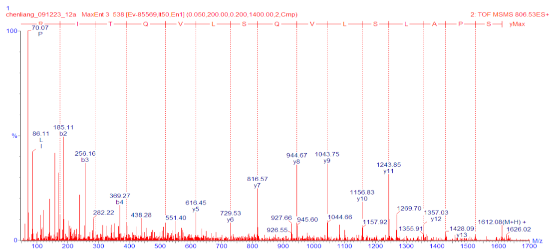
図 58. SPALSLVQSLVQTIR の 2 級質量スペクトル
