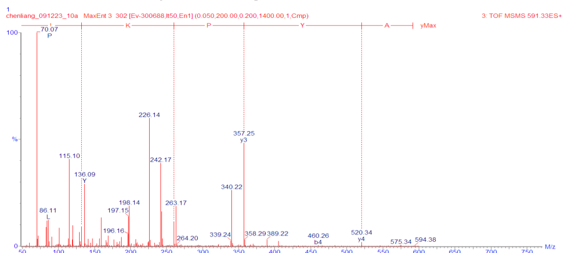
図 45 . AYPKI の 2 級質量スペクトル
