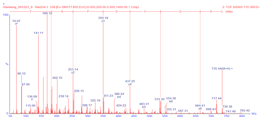
図 35. AQVSPAY の 2 級質量スペクトル
