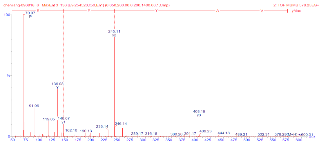
図 25. VAYPE の 2 級質量スペクトル
