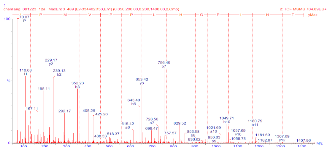
図 57. THIPGHLPPVMPI の 2 級質量スペクトル
