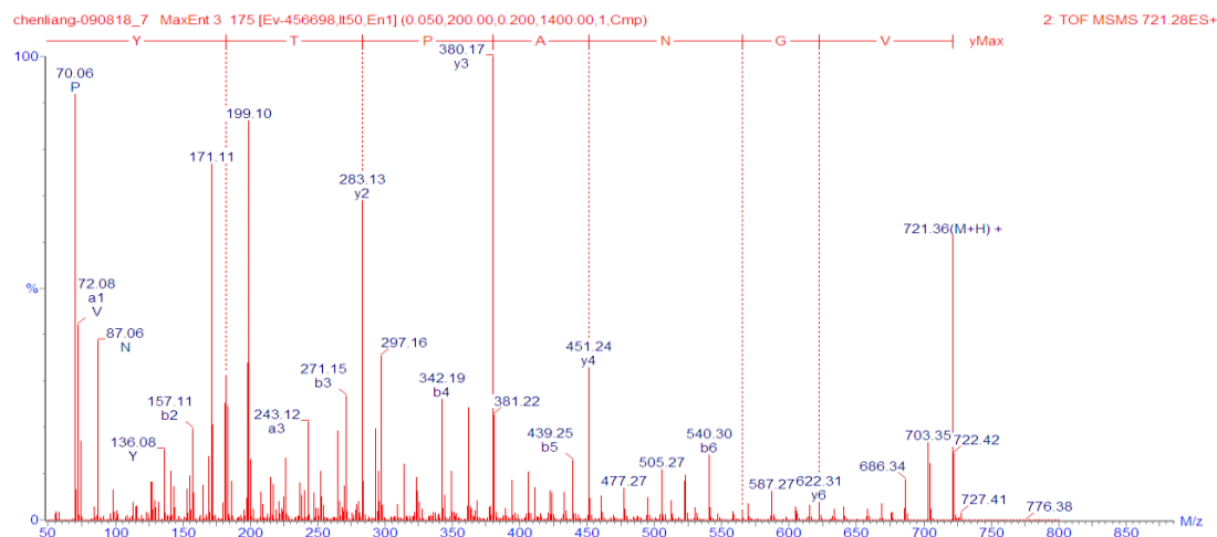
図 28. VGNAPTY の 2 級質量スペクトル
