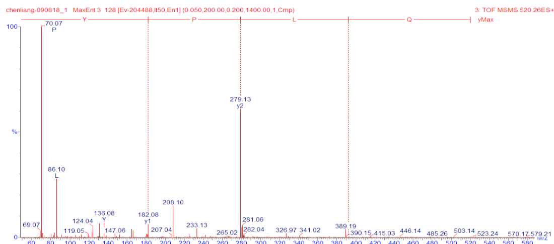
図 6. QLPY の 2 級質量スペクトル
