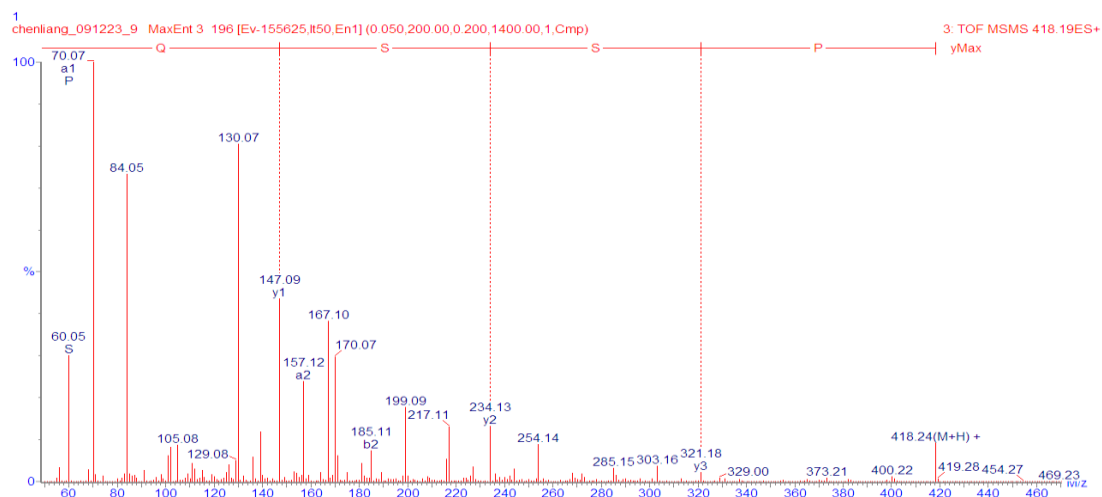
図 34. PSSQ の 2 級質量スペクトル
