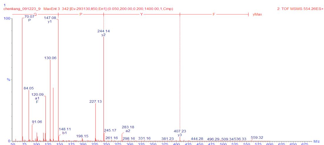
図 38. FYPQ の 2 級質量スペクトル
