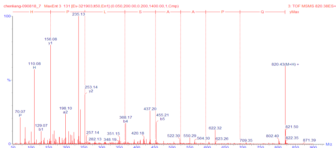
図 30. QPAASLPH の 2 級質量スペクトル
