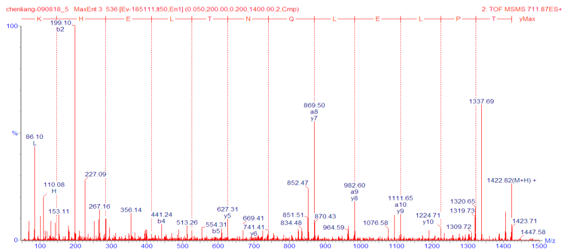
図 22. TPLELQNTLEHK の 2 級質量スペクトル
