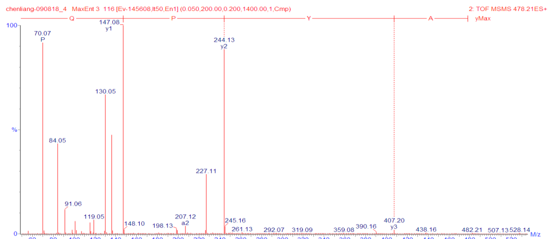
図 16. AYPQ の 2 級質量スペクトル
