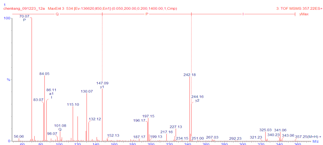
図 54. IPQ の 2 級質量スペクトル
