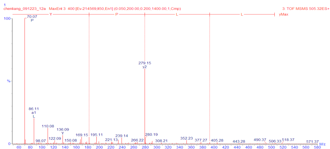
図 55. LLPY の 2 級質量スペクトル
