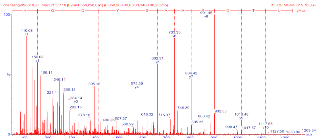
図 40. LTDPAASYQQH の 2 級質量スペクトル
