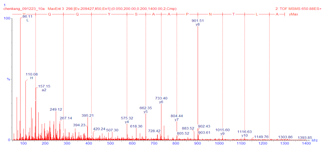
図 44 . ALTNPAAASYQQH の 2 級質量スペクトル
