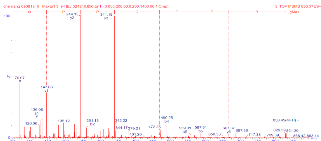
図 27. YPTQPPQ の 2 級質量スペクトル
