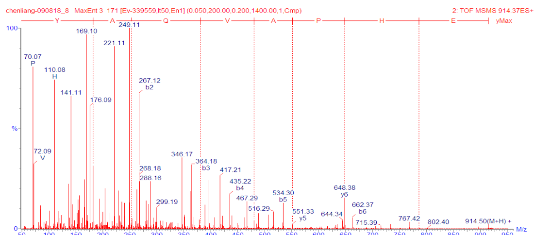
図 39. EHPAVQAY の 2 級質量スペクトル
