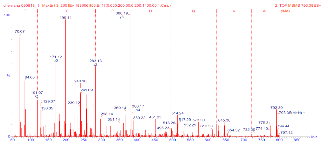
図 5. AVQDPYT の 2 級質量スペクトル
