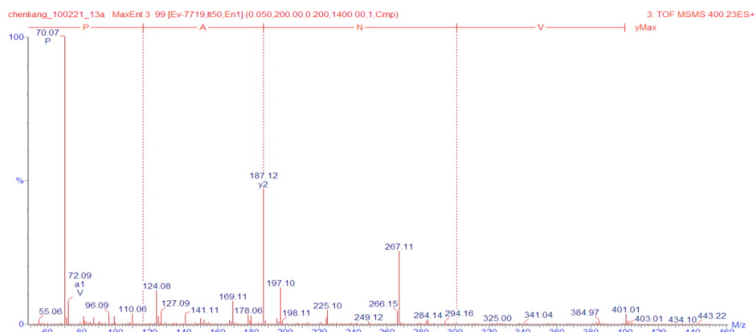
図 15. VNAP の 2 級質量スペクトル
