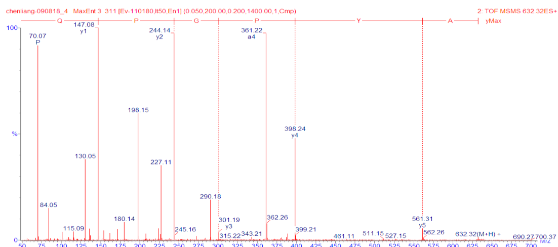
図 18. AYPGPQ の 2 級質量スペクトル
