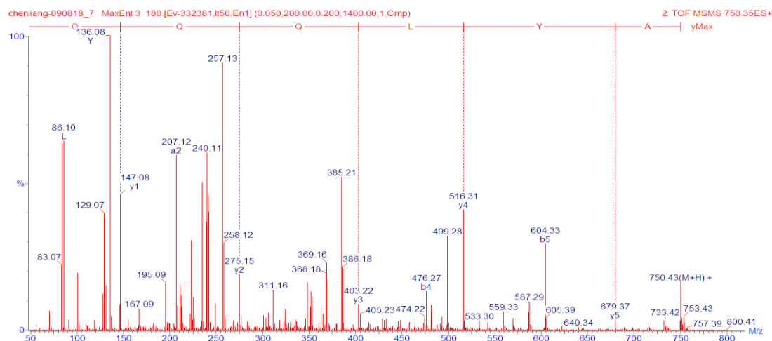
図 29. AYLQQQ の 2 級質量スペクトル
