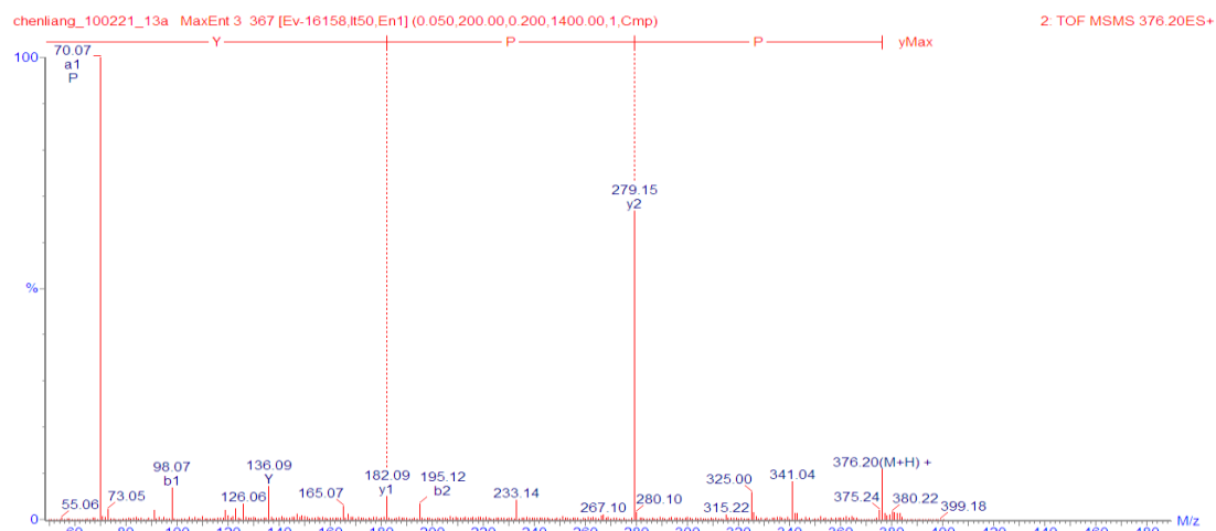
図 14. PPY の 2 級質量スペクトル
