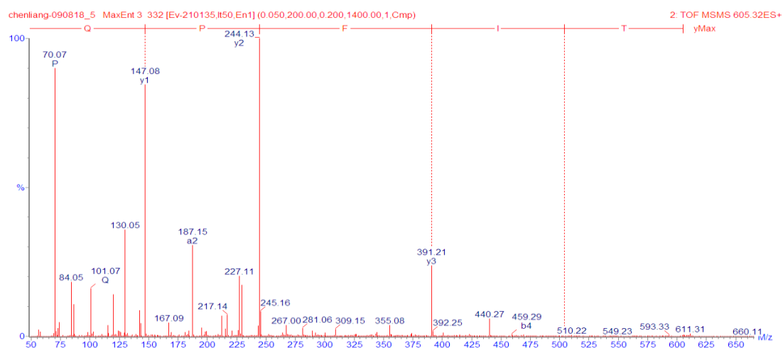
図 20. TIFPQ の 2 級質量スペクトル
