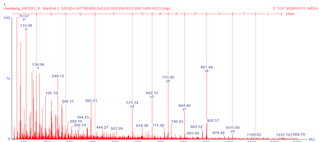
図 37. LTNPAASYQQH の 2 級質量スペクトル
