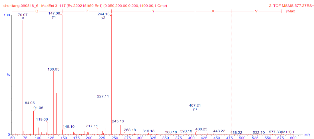
図 24. VAYPQ の 2 級質量スペクトル
