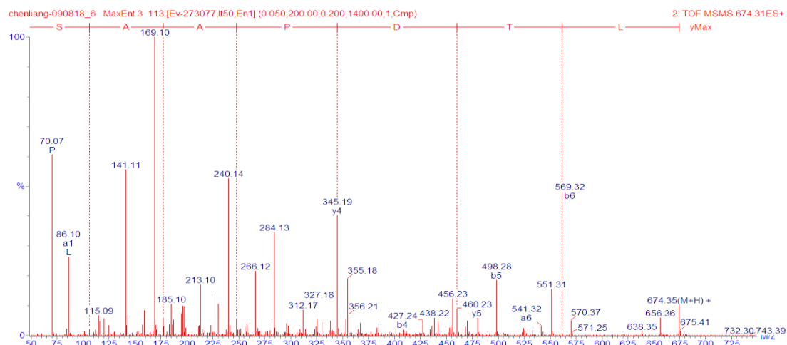
図 26. LTDPAAS の 2 級質量スペクトル
