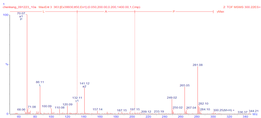
図 47. PAL の 2 級質量スペクトル
