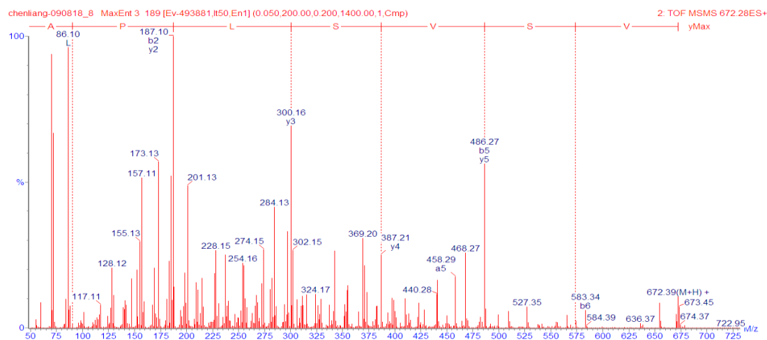
図 41. VSVSLPA の 2 級質量スペクトル
