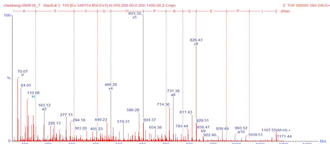
図 31. LPEGAPHGVYK の 2 級質量スペクトル
