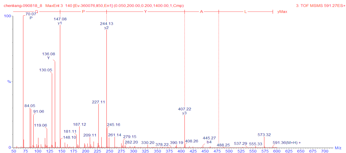
図 43. LAYPQ の 2 級質量スペクトル
